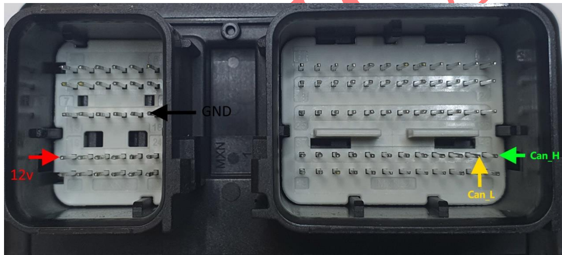
a) 气囊电控单元接线说明 飞线和引脚说明
