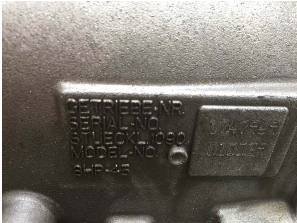
图 1：波箱型号 8HP-45
