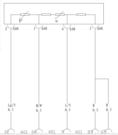
进气总管温度压力传感器
