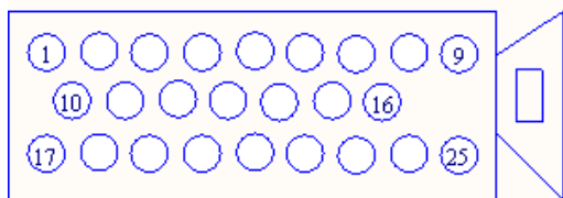
引脚排列示意图：
