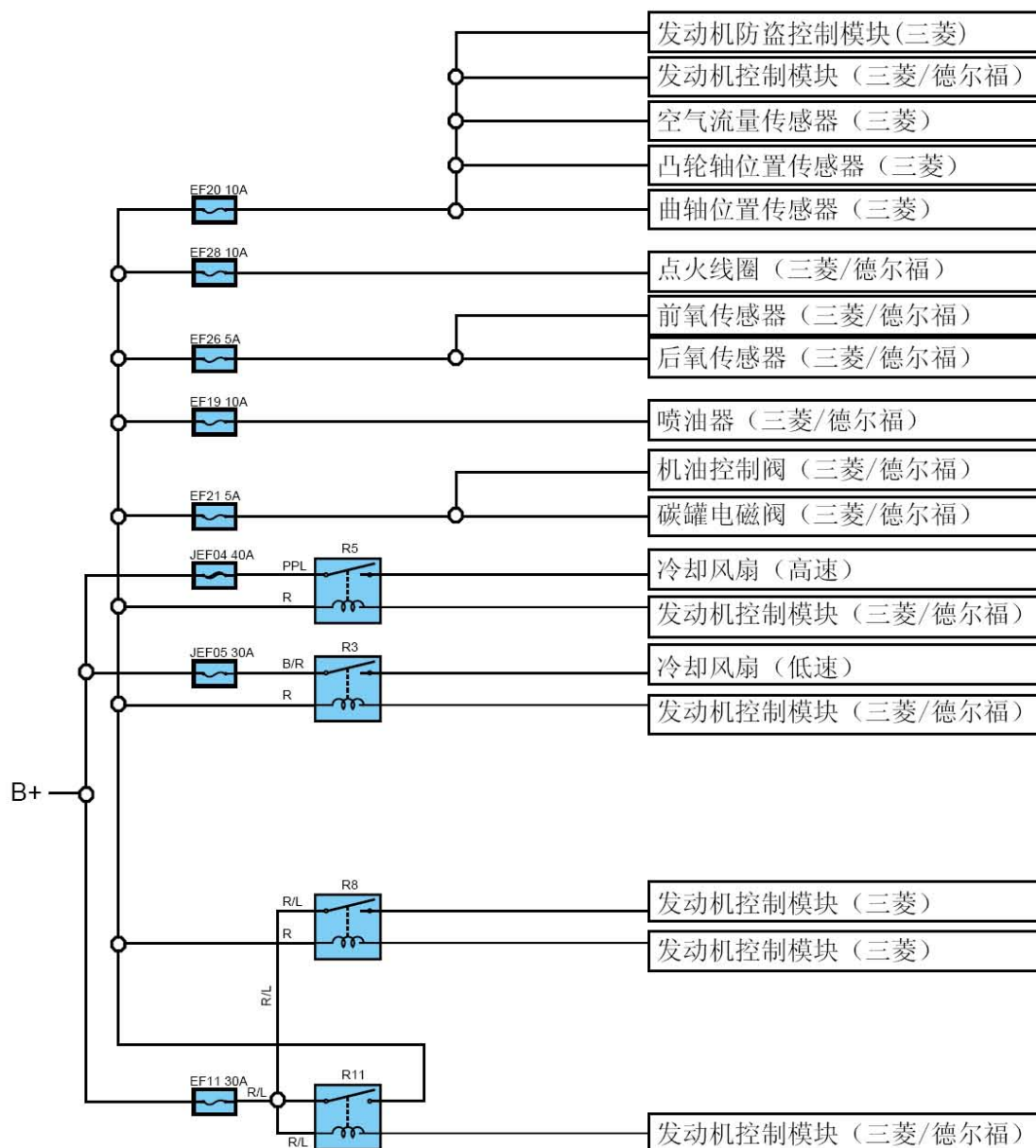
附：保险丝、继电器及用电器控制分布图
