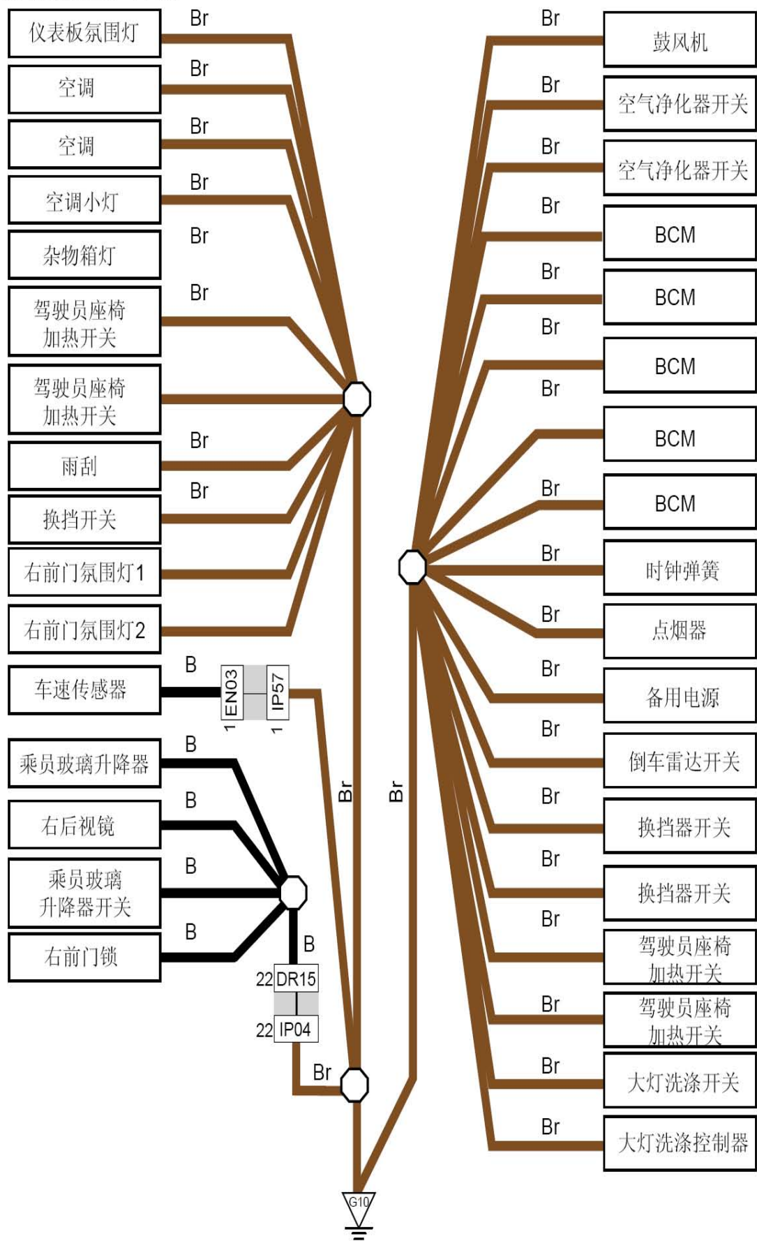
接地线路图6 (G10)
