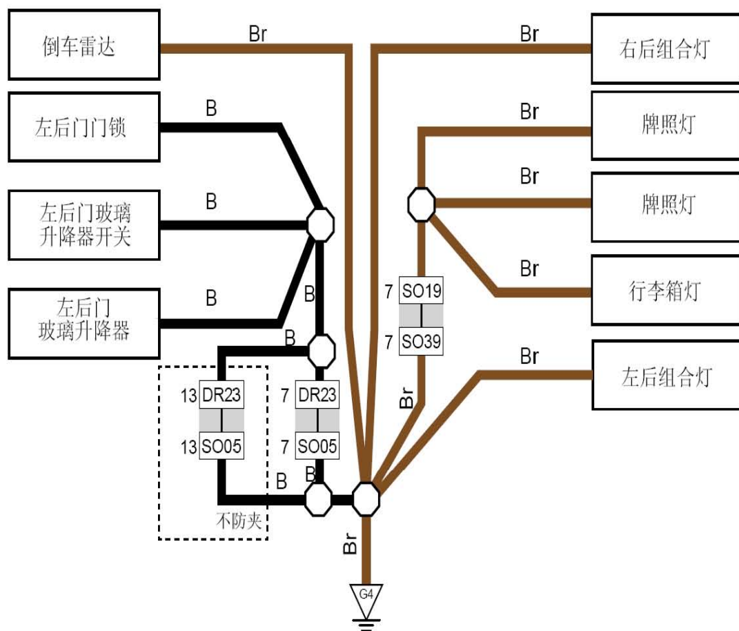
接地线路图3 (G4, G6)
