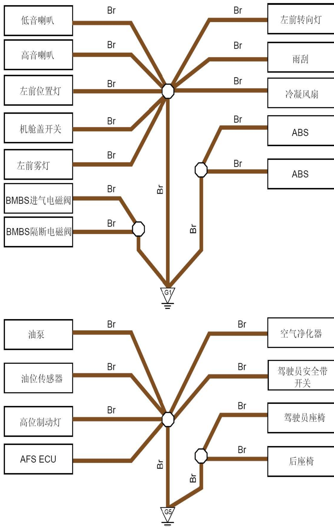
接地线路图1 (G1、G5)
