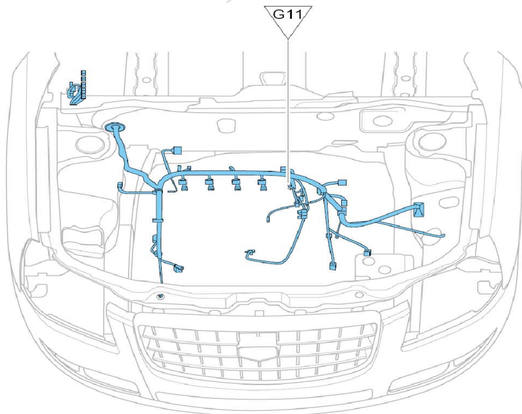
发动机舱接地点布置图(续)
