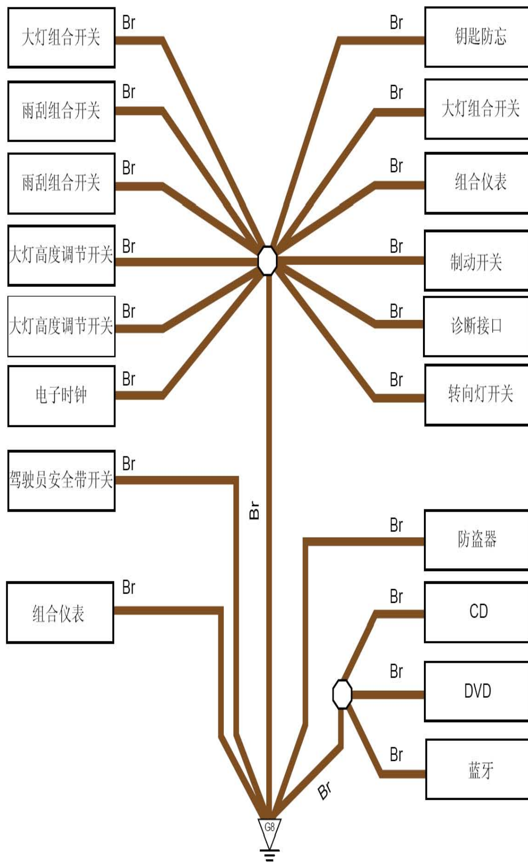
接地线路图5 (G8)
