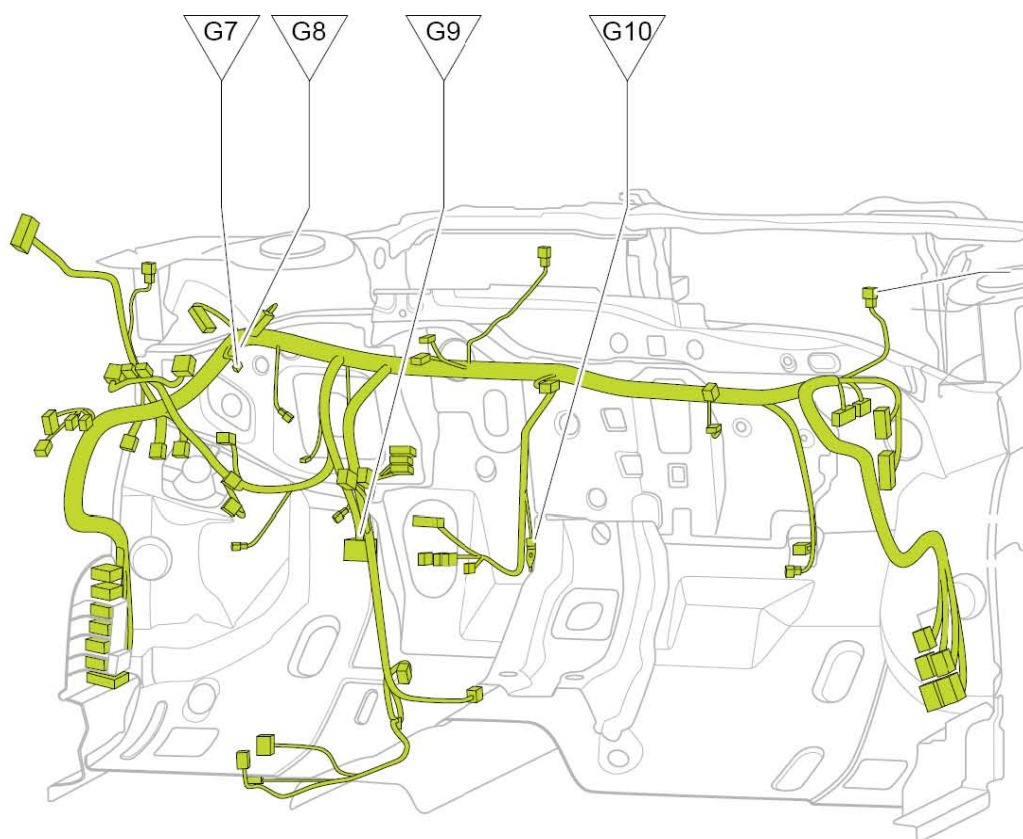
仪表板接地点布置图
