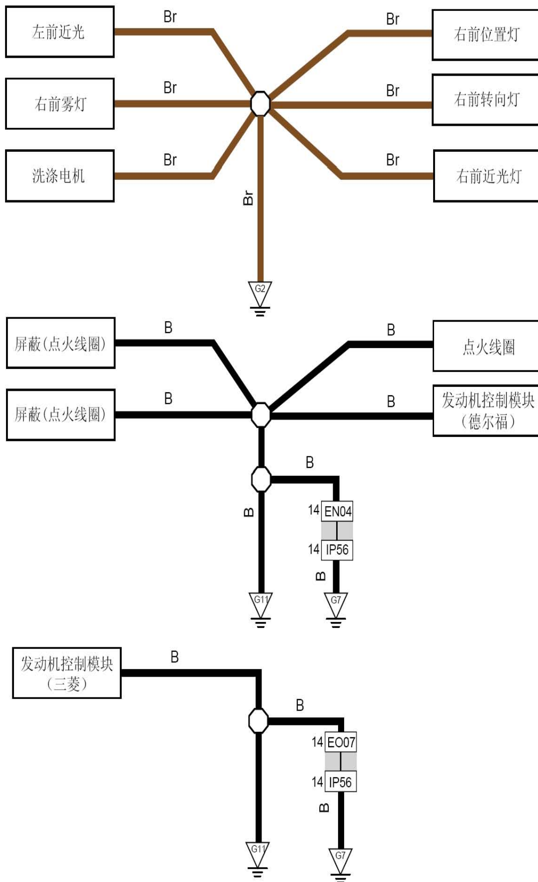
接地线路图7 (G2、G7、G11)
