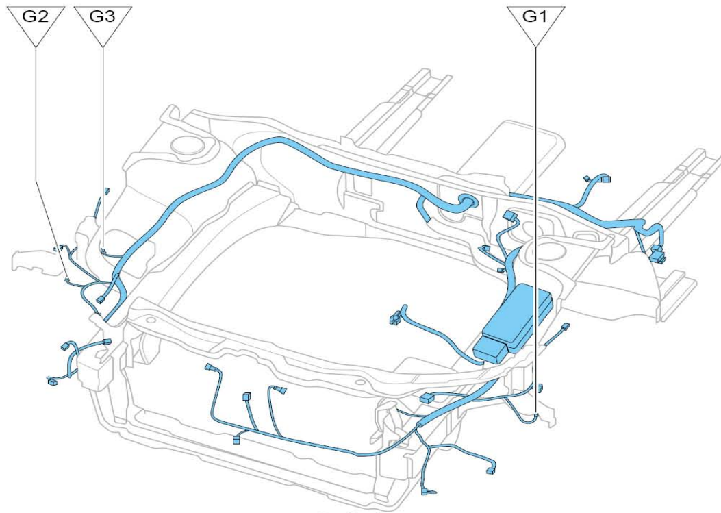
发动机舱接地点布置图
