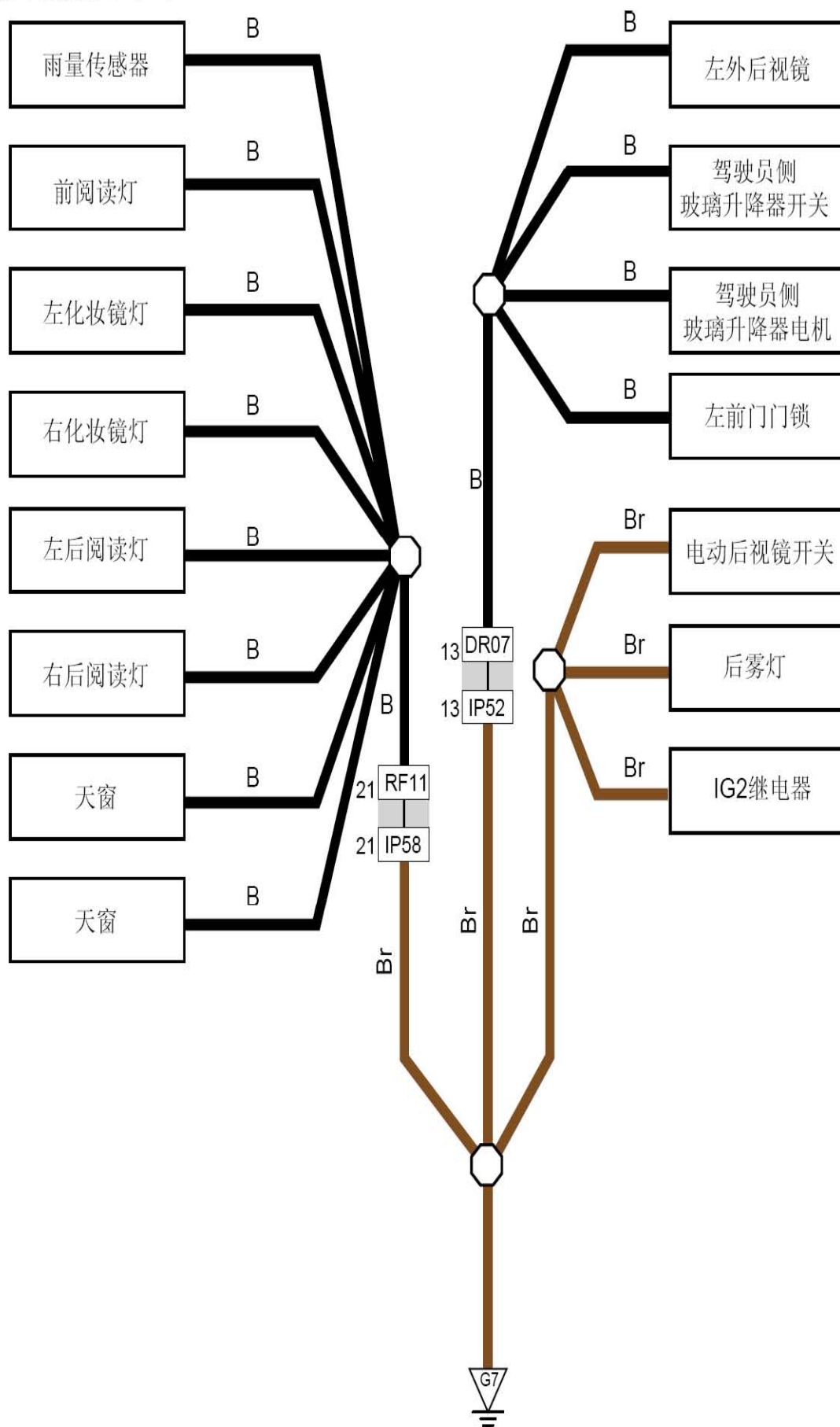
接地线路图4 (G7)
