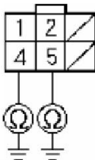
凹头插头导线侧
