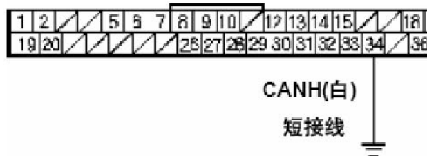
凹头插头导线侧
