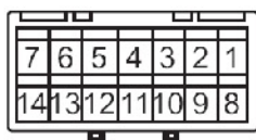
乘员侧侧气帘线束连接器 RF03
