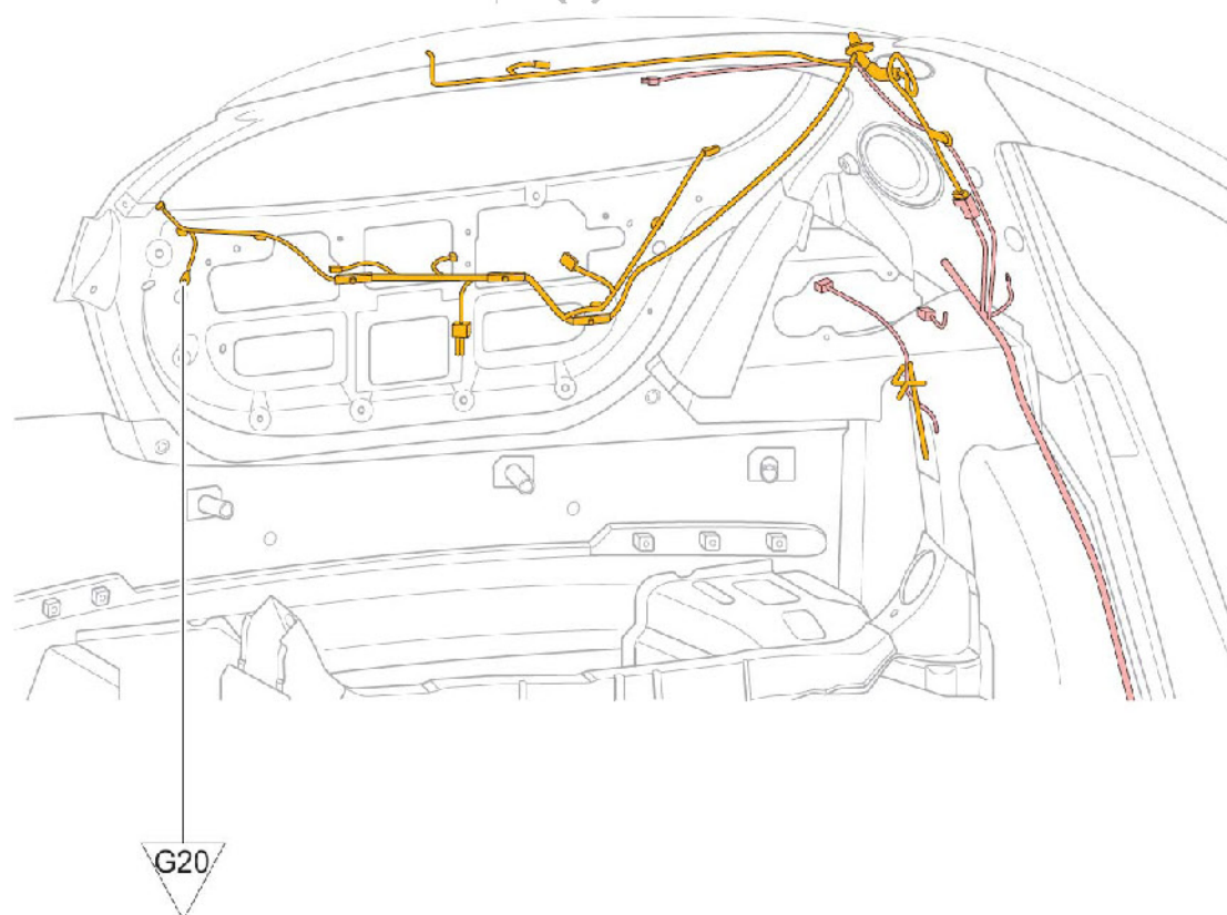
背门接地点布置图(两厢)
