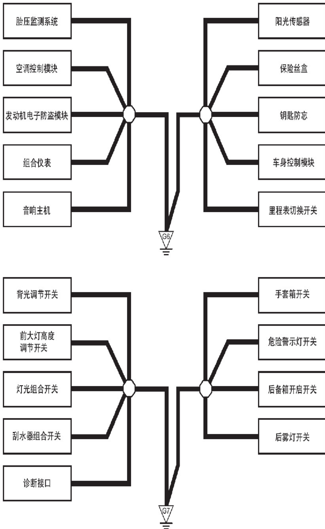
接地线路图1 (G6、G7)
