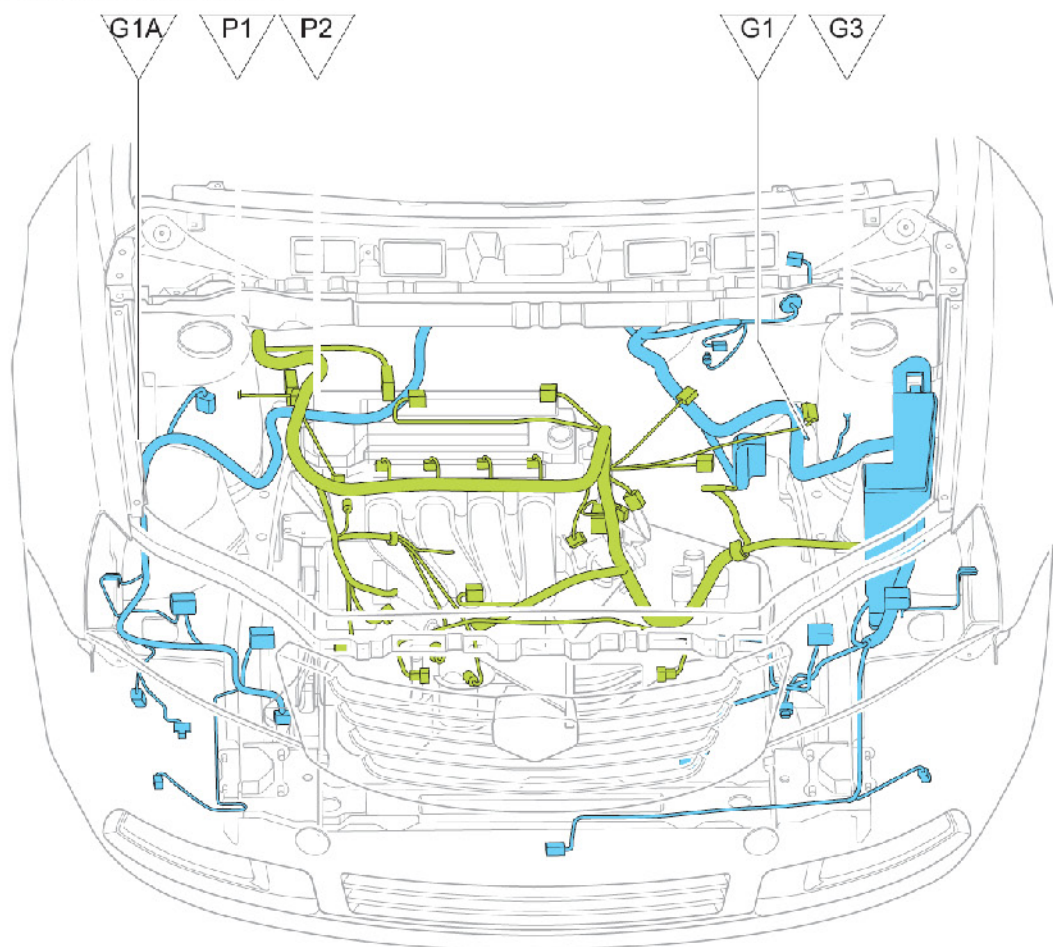
发动机舱接地点布置图
