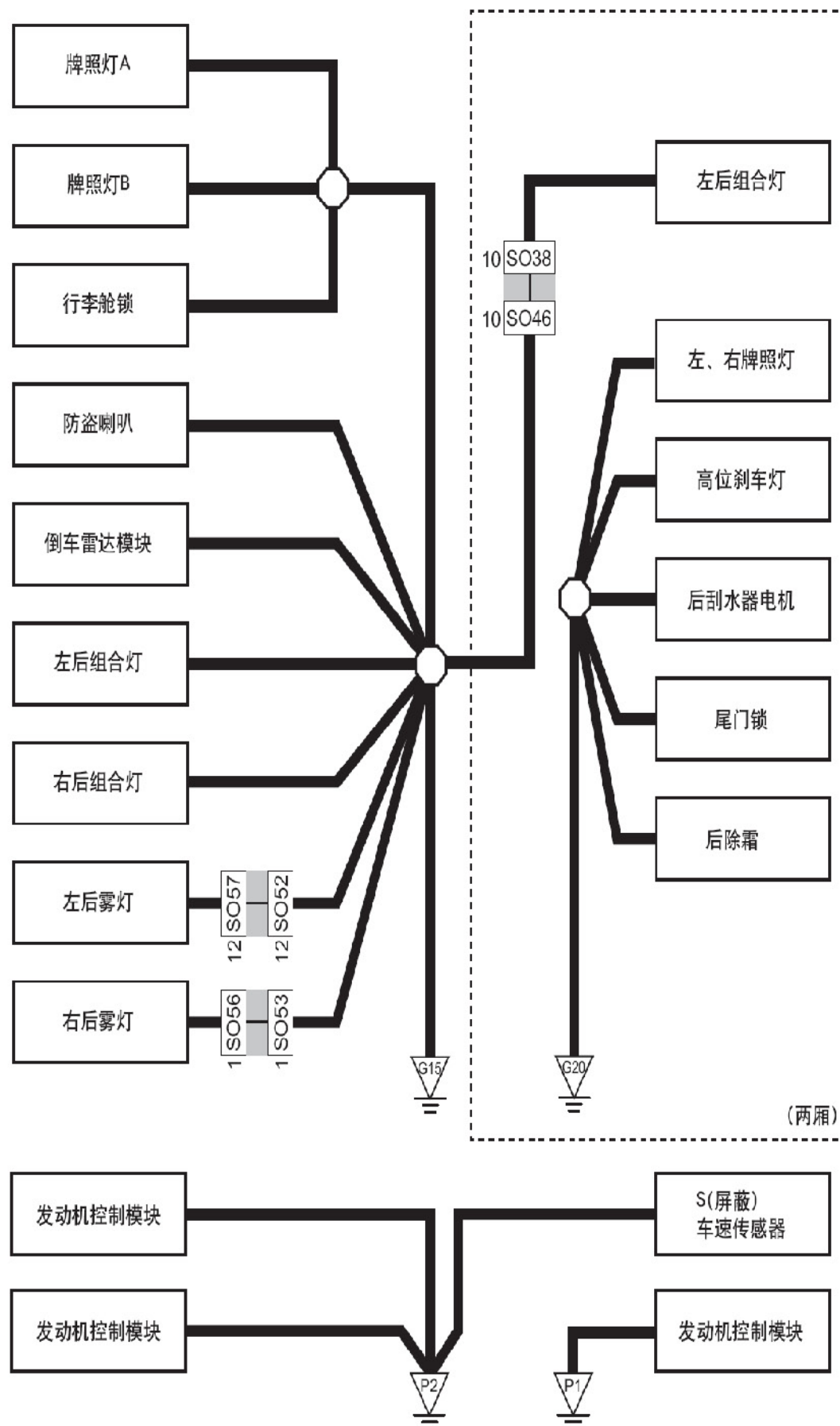
接地线路图5 (G15, G20, P1, P2)
