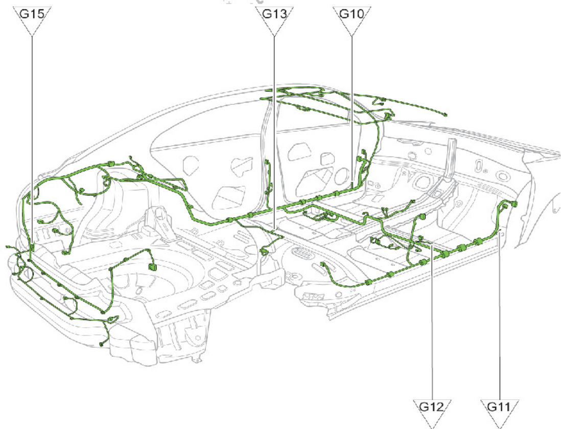
底板接地点布置图(三厢)
