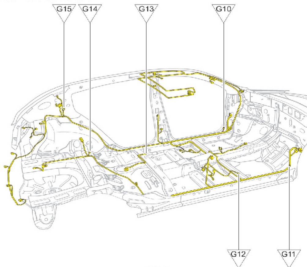
底板接地点布置图(两厢)
