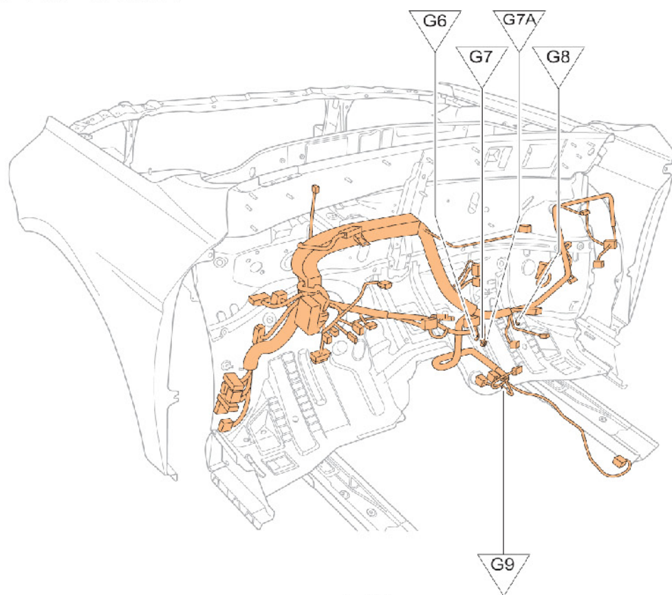
仪表板接地点布置图
