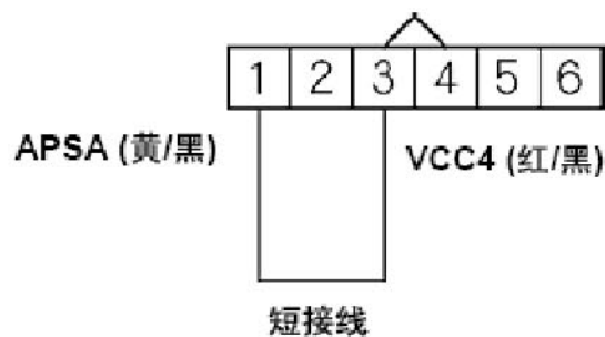
凹头插头导线侧
