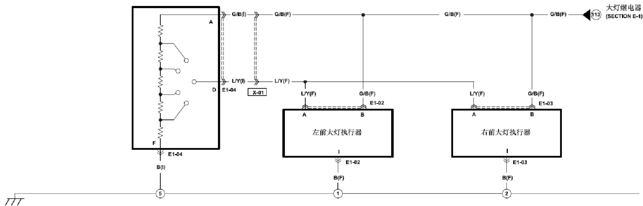
大灯调节开关
