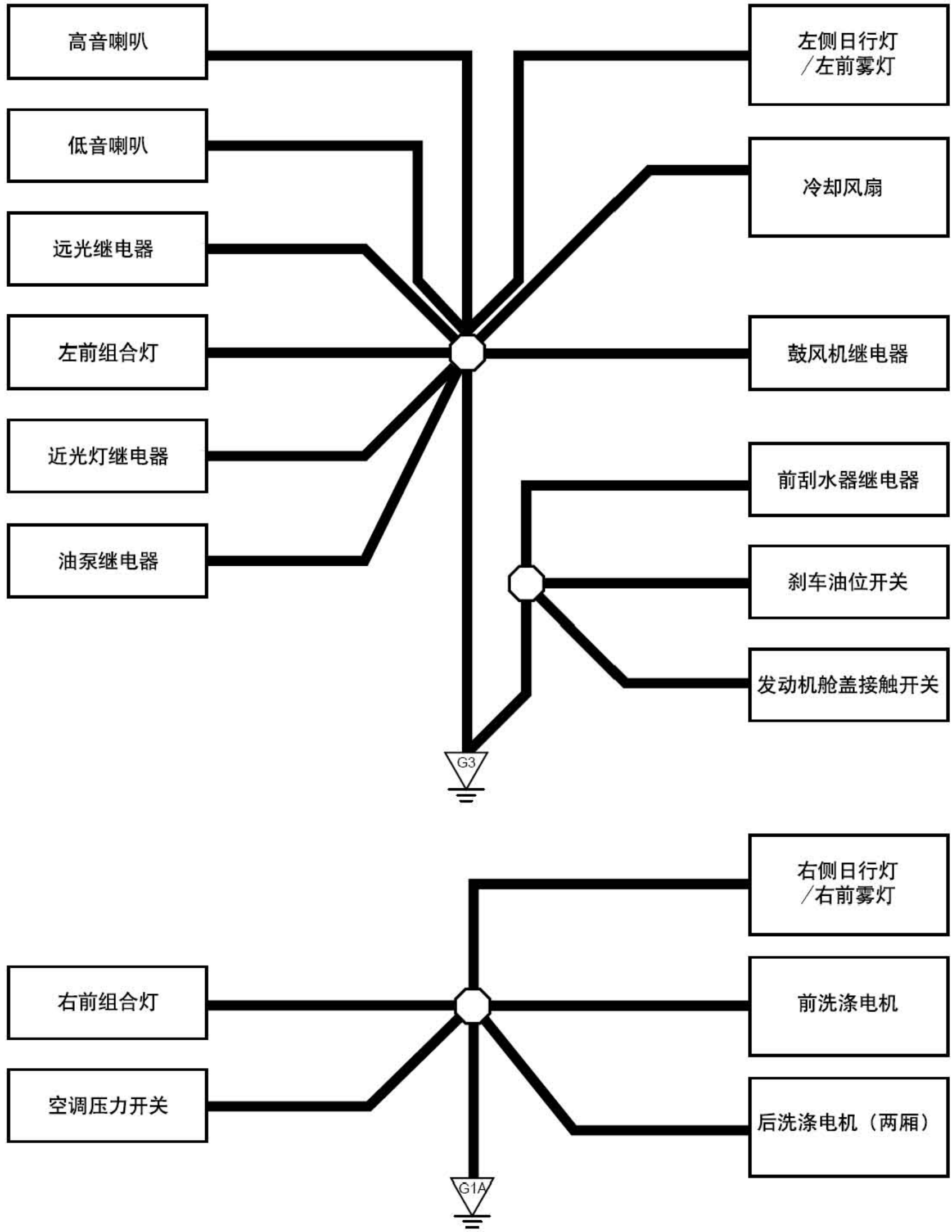
接地线路图5 (G1A, G3) (JL4G15-G)
