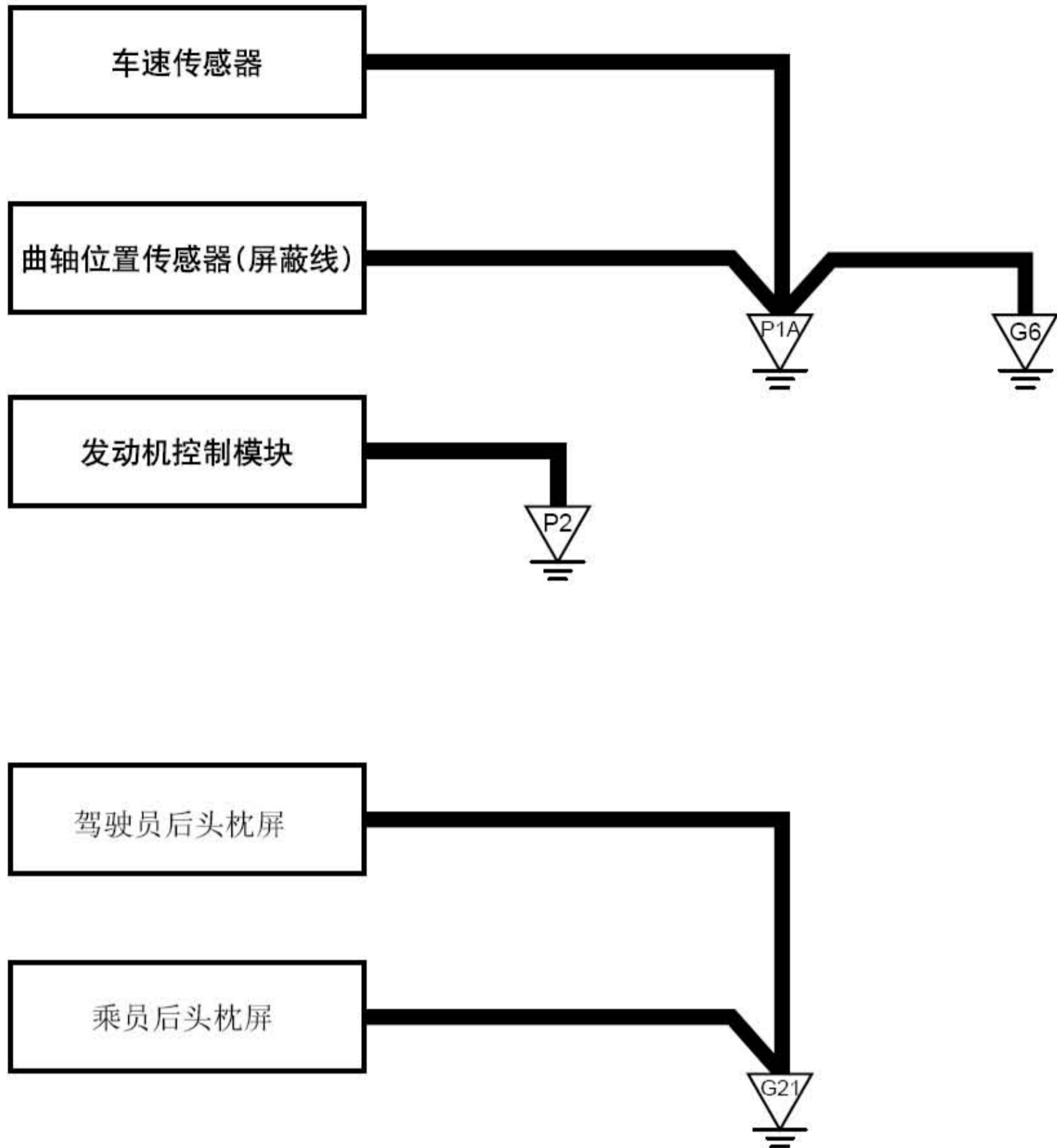
接地线路图7 (P1A、P2、G6)
