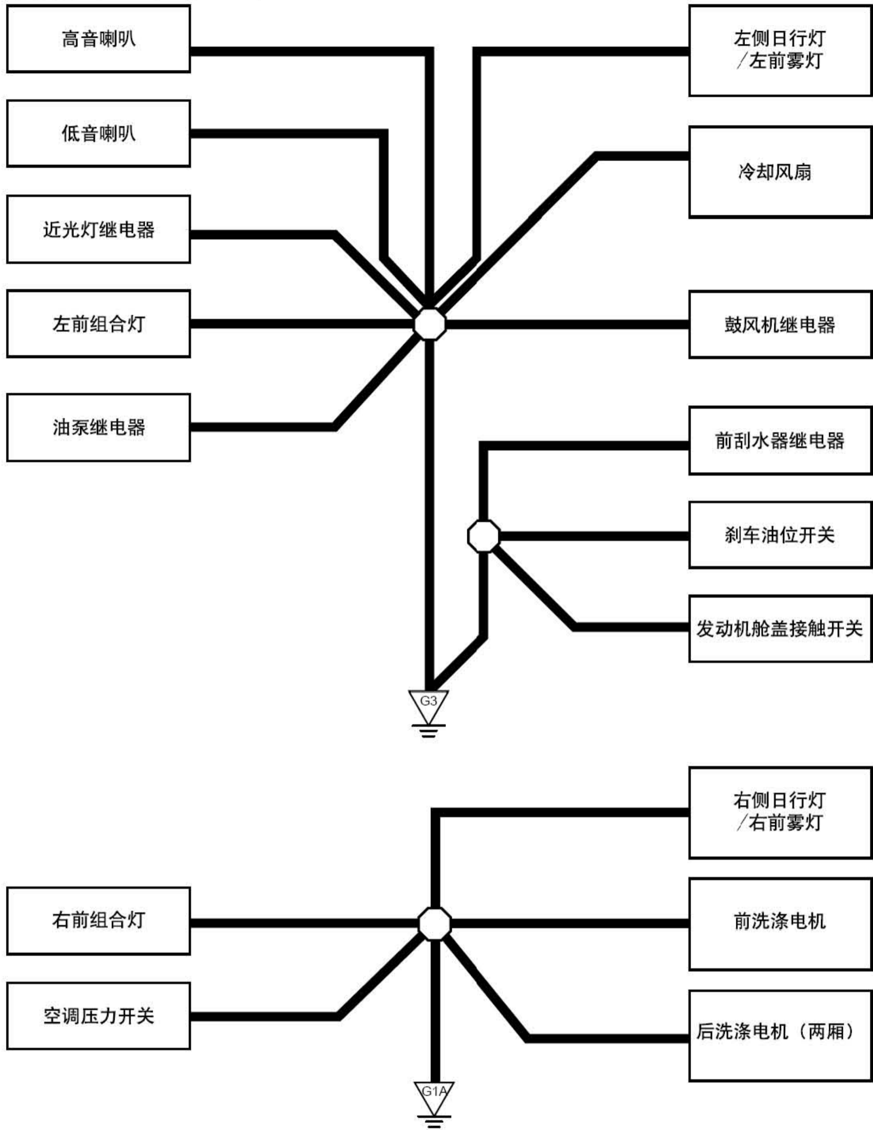
接地线路图6 (G1A、G3) (JL4G15-G)
