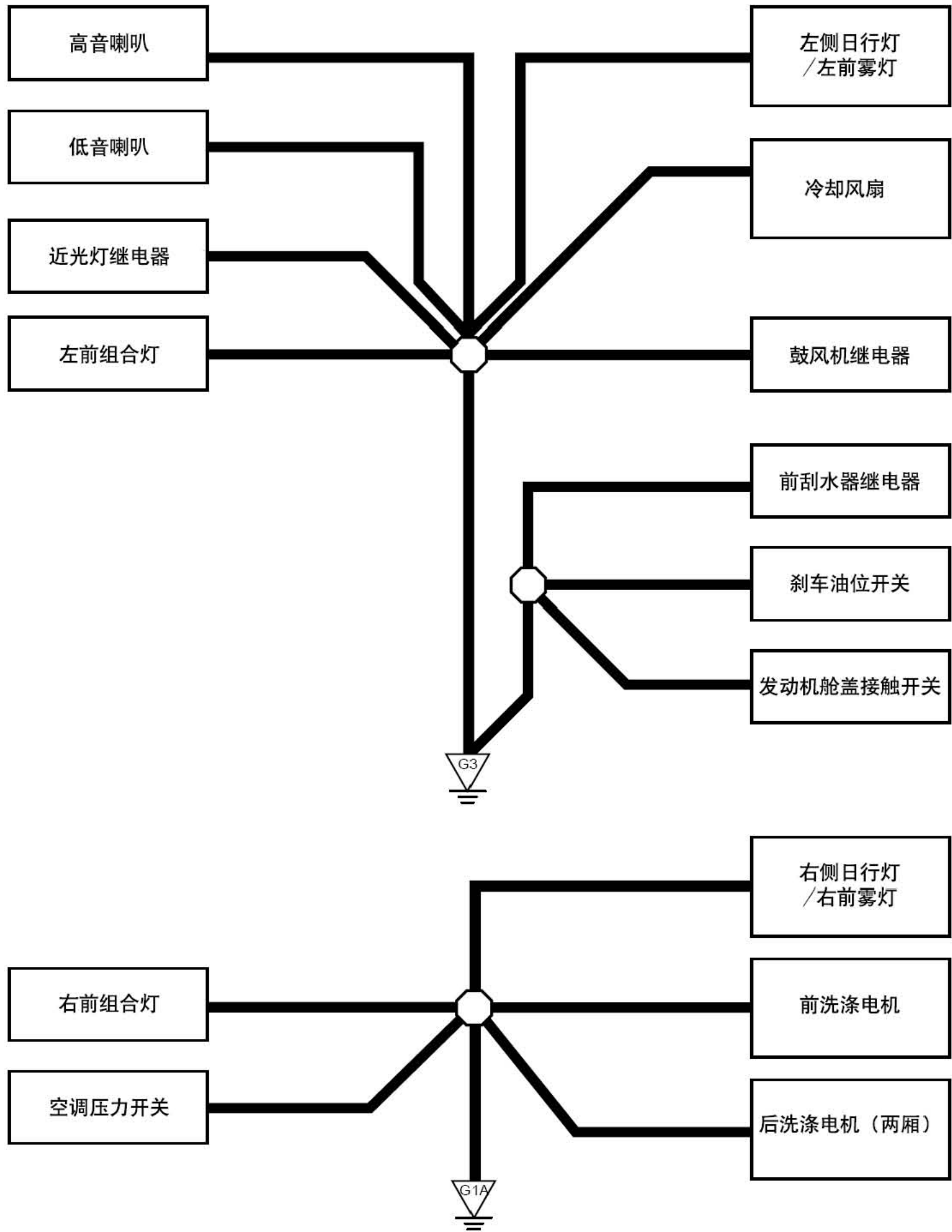
接地线路图4 (G1A、G3)
