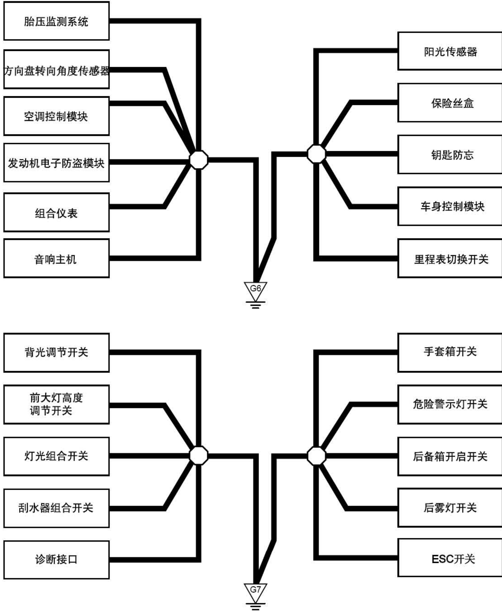
接地线路图1 (G6、G7)
