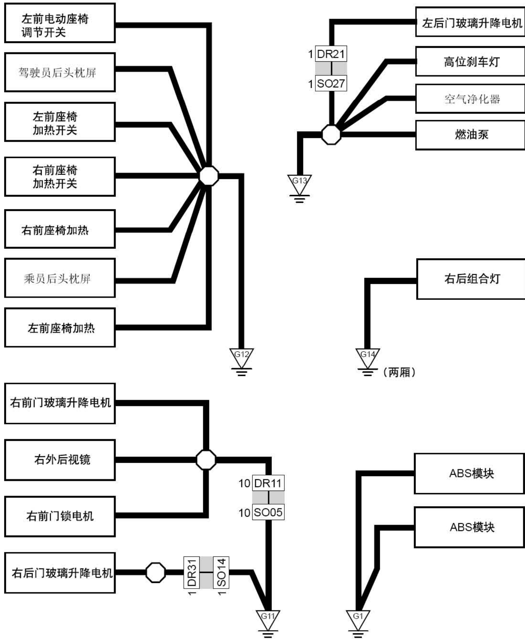
接地线路图2 (G1、G11、G12、G13、G14)
