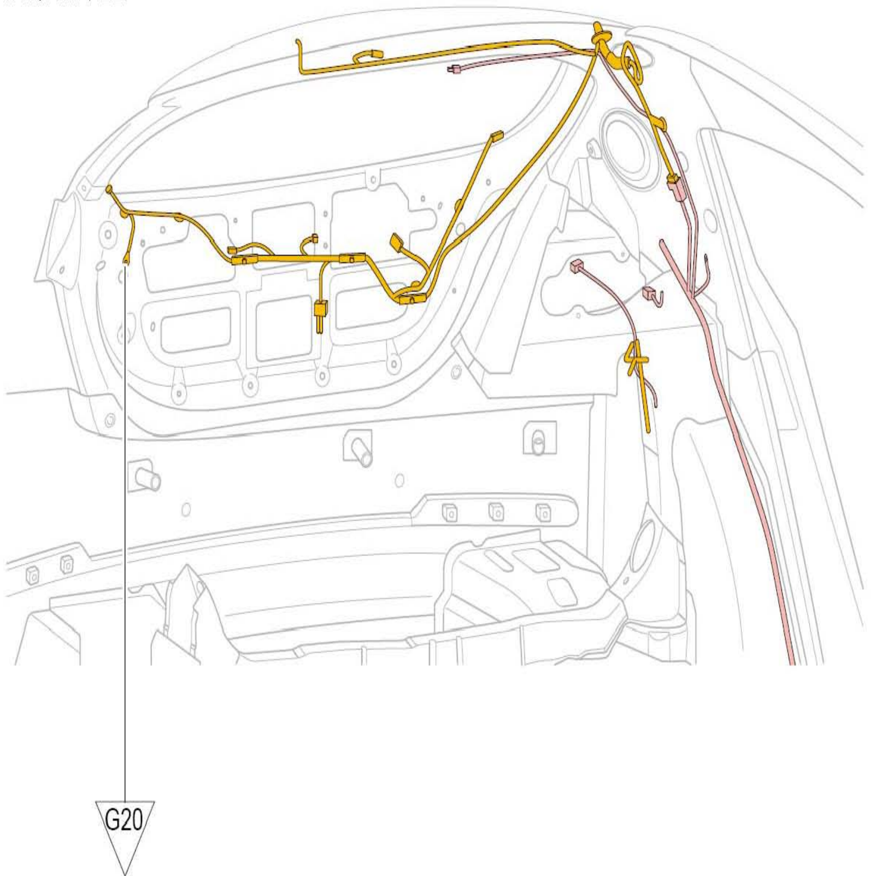
背门接地点布置图
