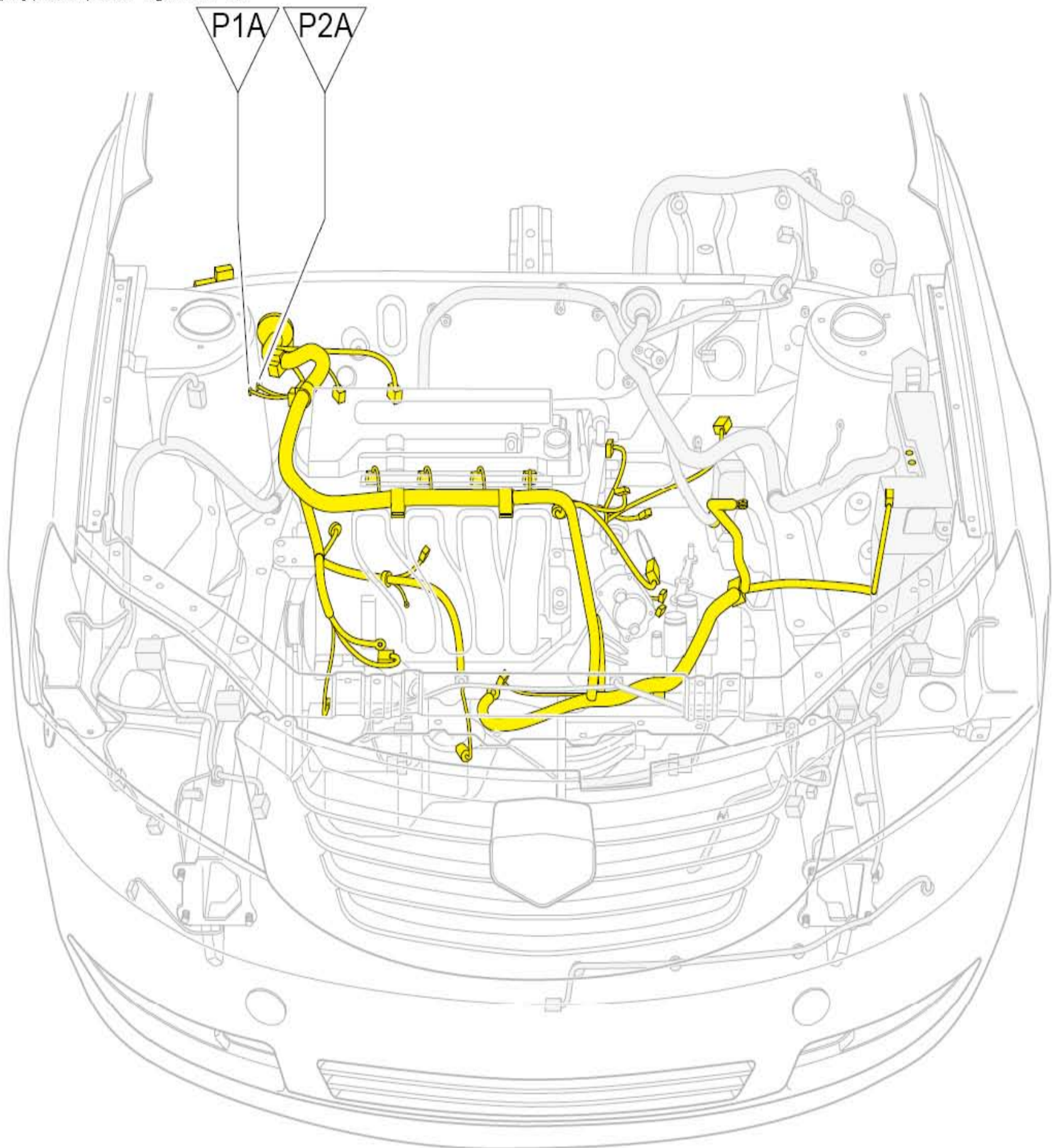
发动机接地点布置图 (JL4G15-G)
