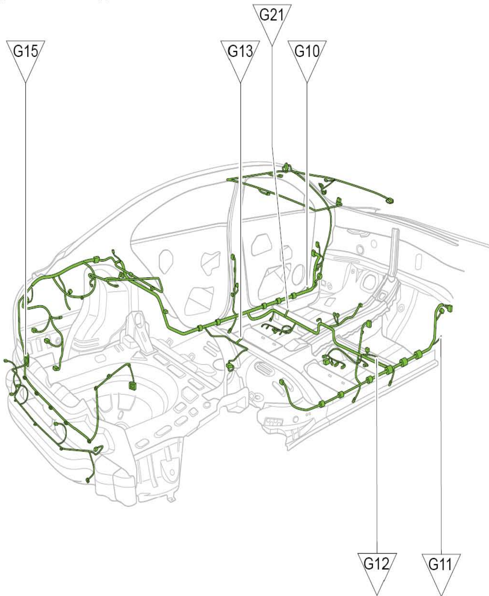
底板接地点布置图（三厢，行政版）
