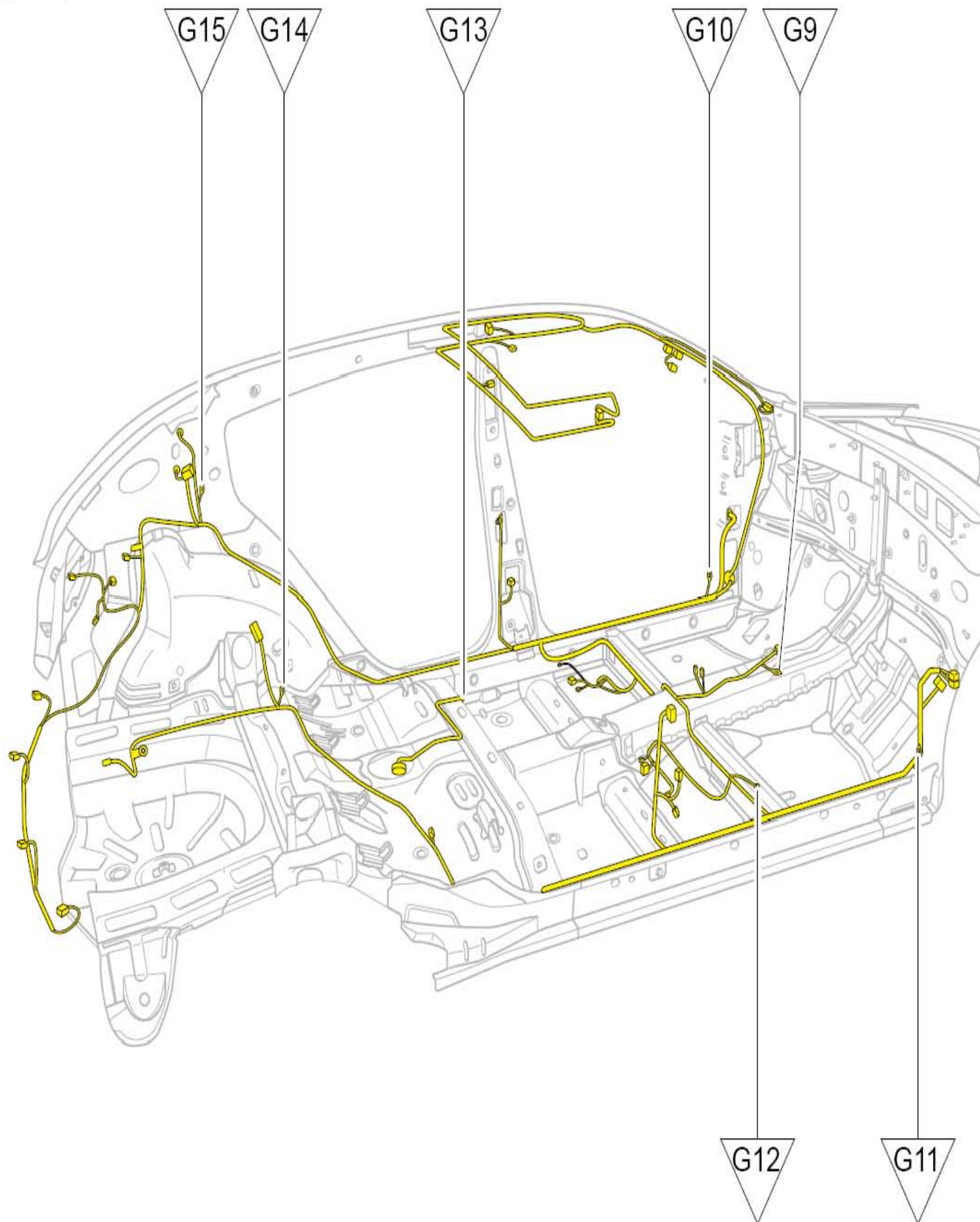
底板接地点布置图（两厢）
