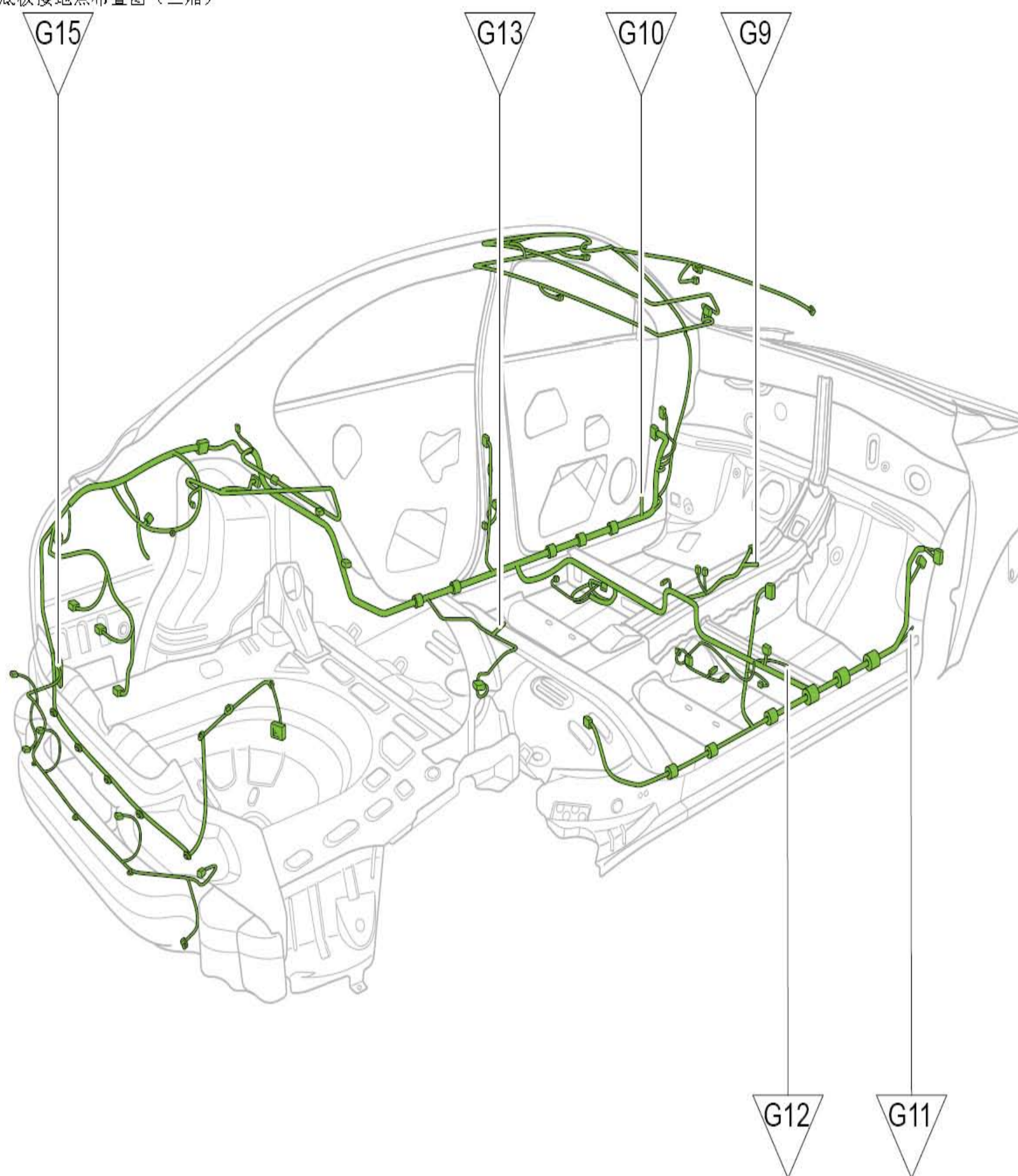
底板接地点布置图（三厢）
