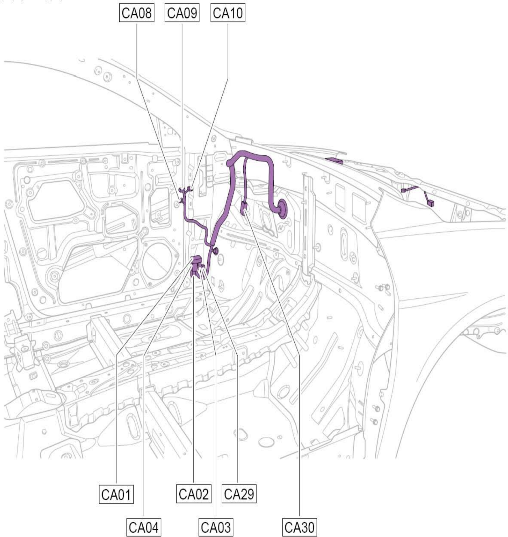
发动机舱线束布置图
