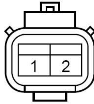
CA29 隔断电磁阀线束连接器
