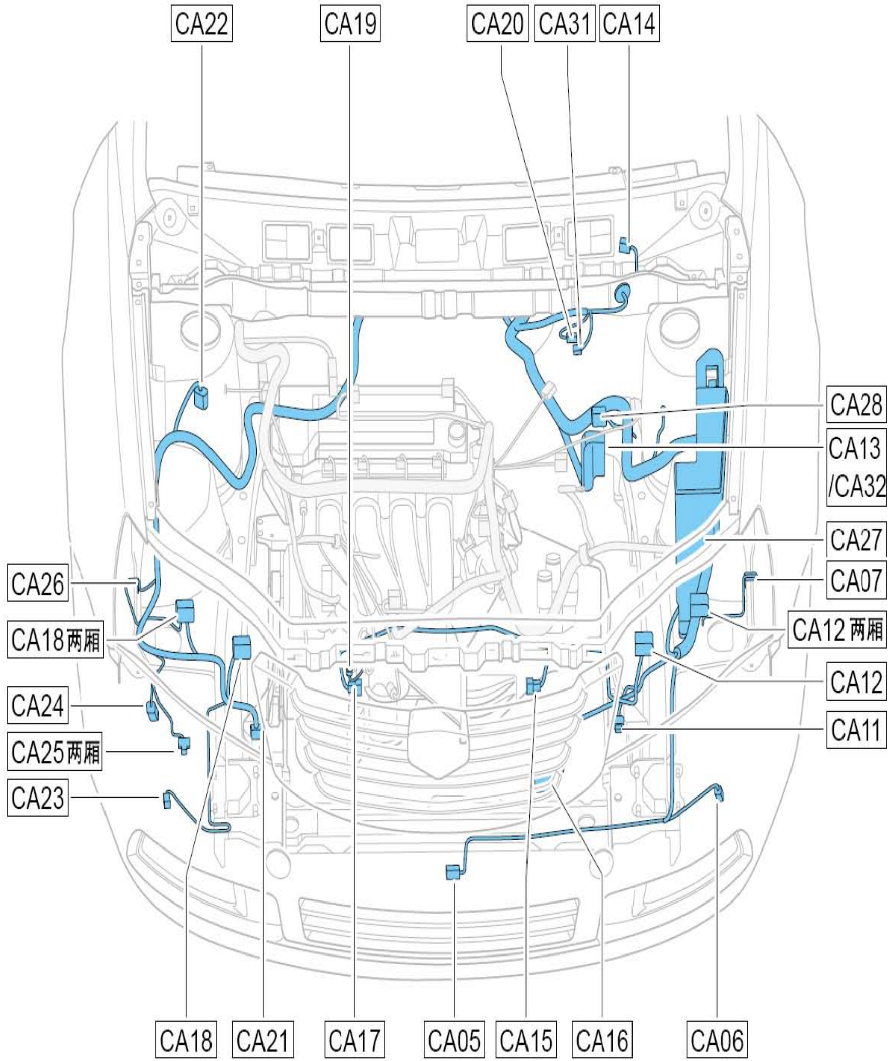
发动机舱线束布置图 (续)
