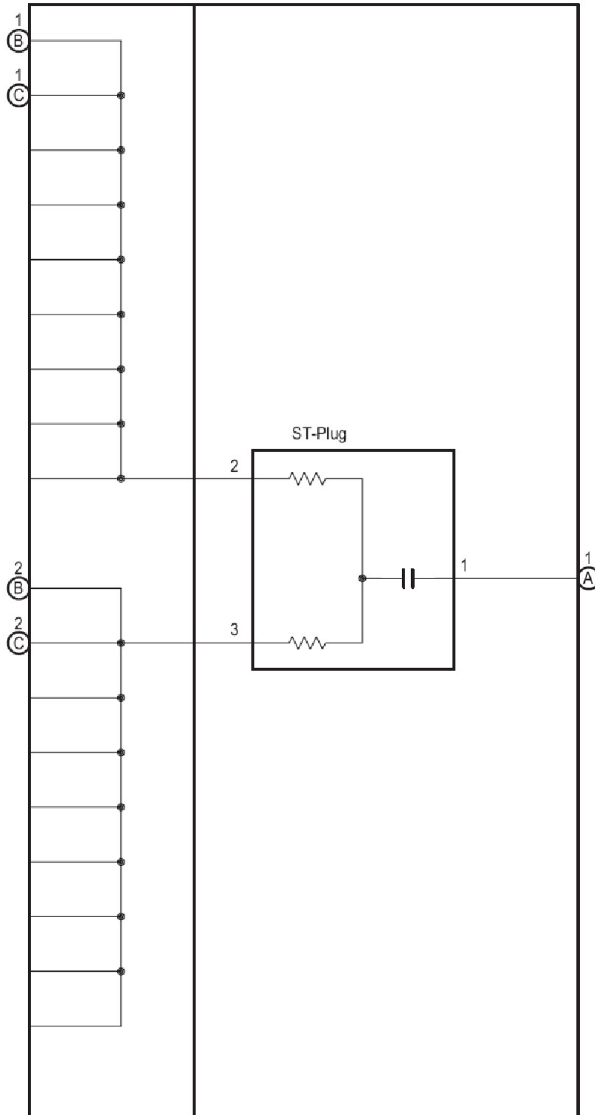
E100(A), E101(B), E102(C) 接线连接器
