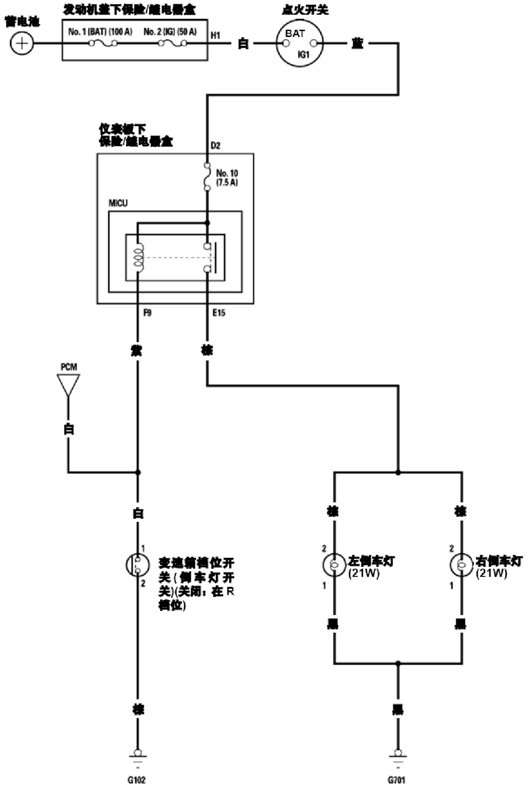
电路图 (续)
