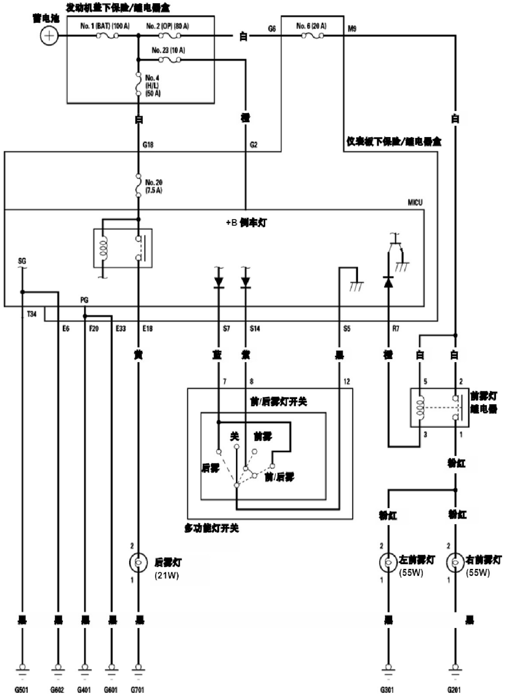
电路图 (续)
