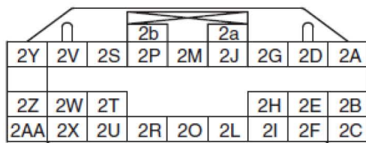
SAS控制模块线束侧连接器
