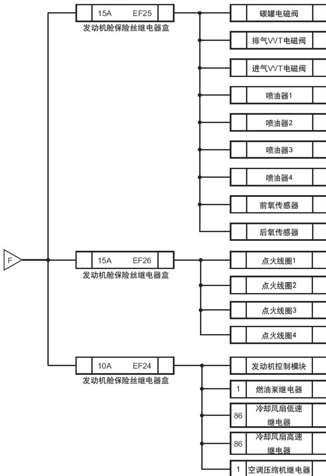
电源配置电路图6
