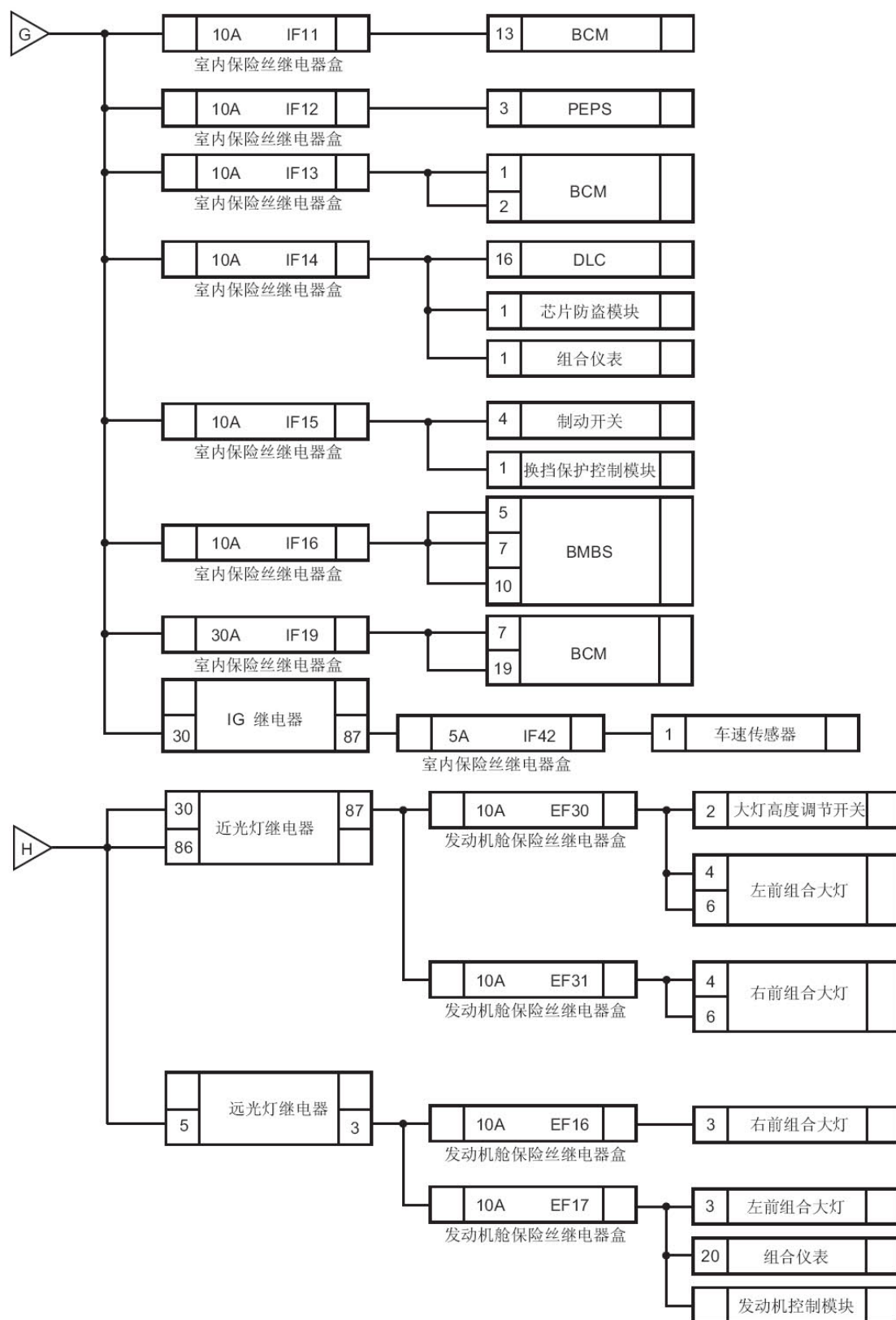
电源配置电路图5
