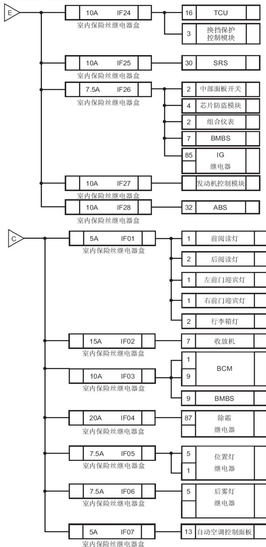
电源配置电路图3
