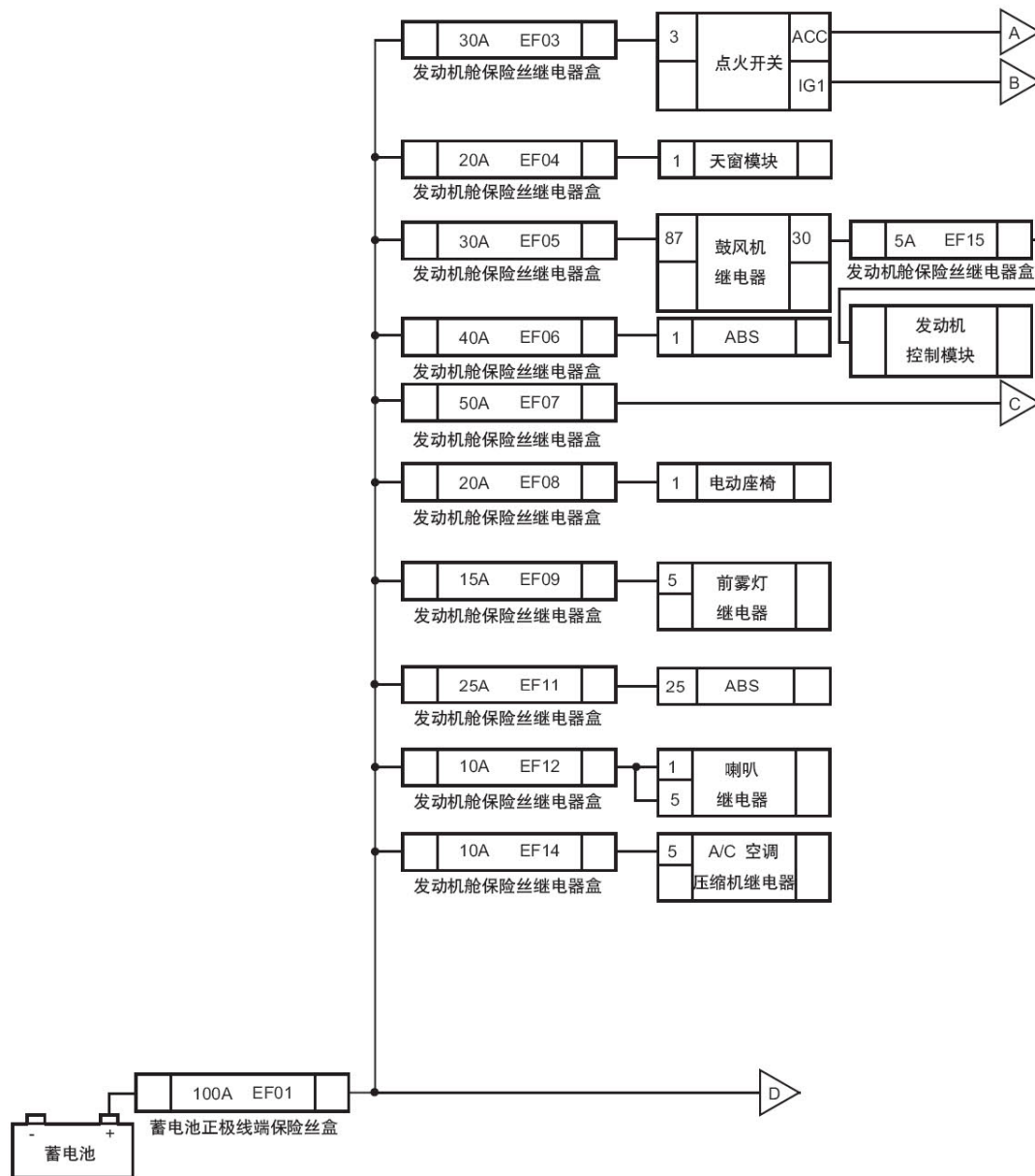
电源配置电路图1
