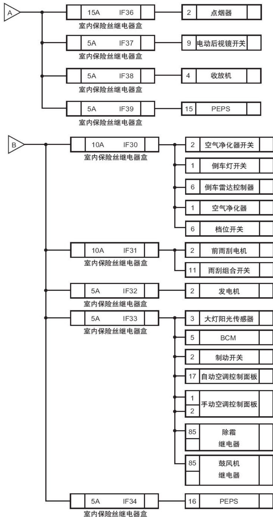
电源配置电路图2
