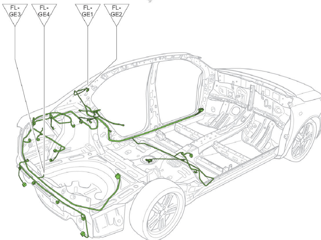
底板接地点布置图
