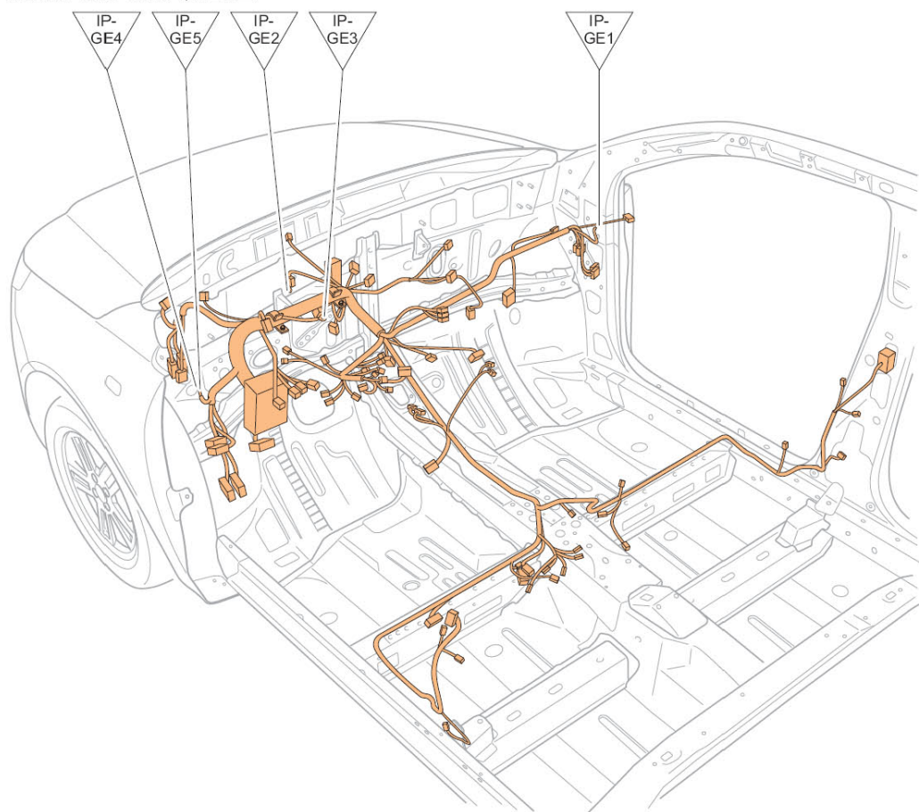
仪表板接地点布置图
