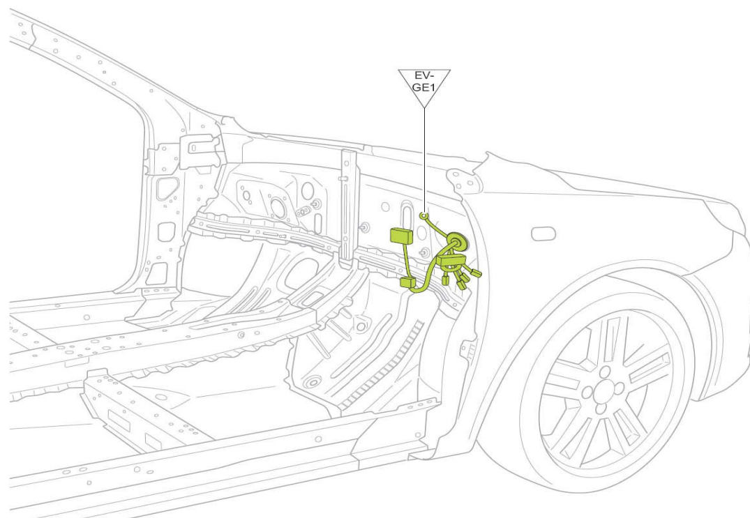
发动机接地点布置图(4G18N-DSI)
