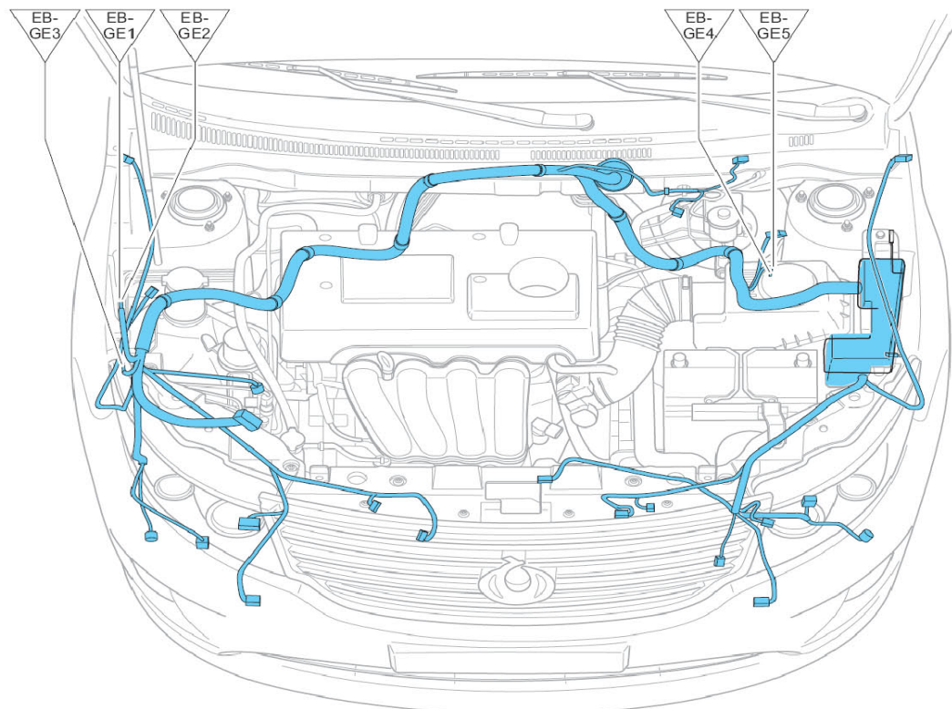
发动机舱接地点布置图
