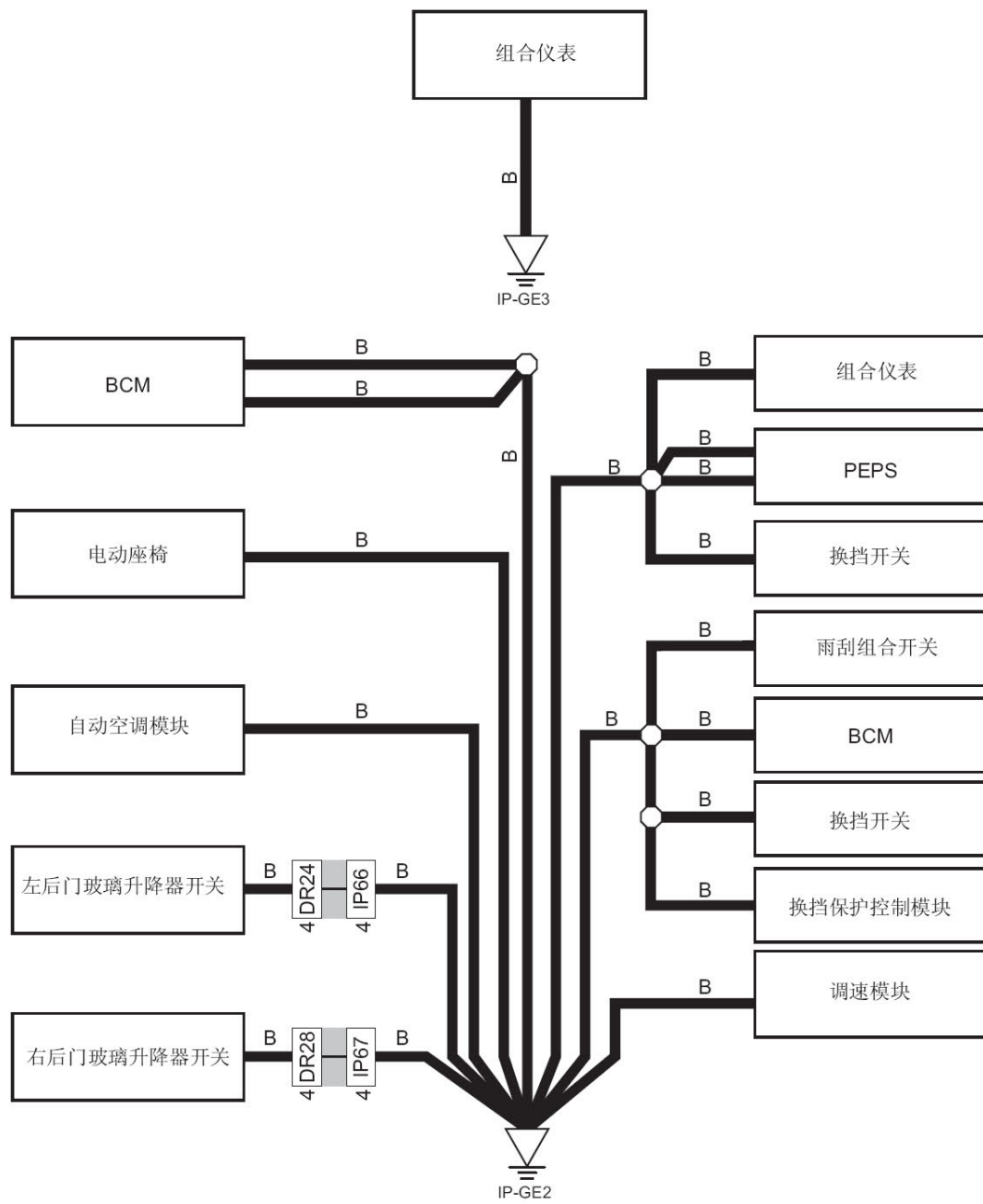
接地线路图5(IP-GE2, IP-GE3)
