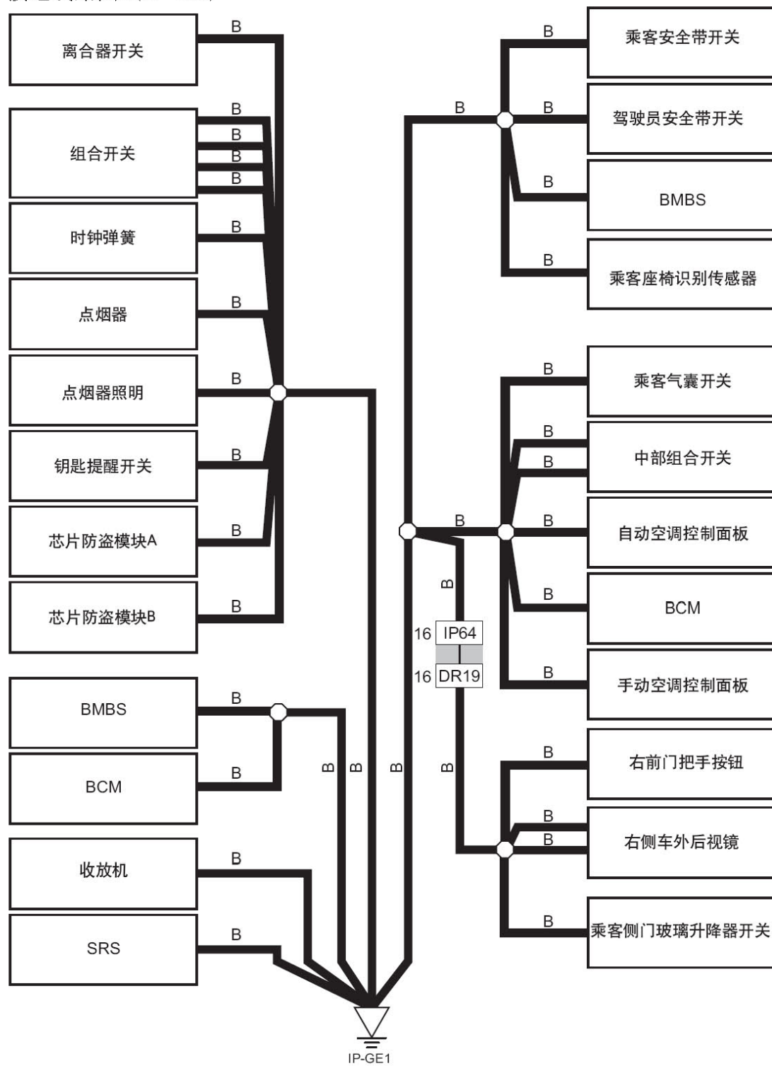
接地线路图4(IP-GE1)
