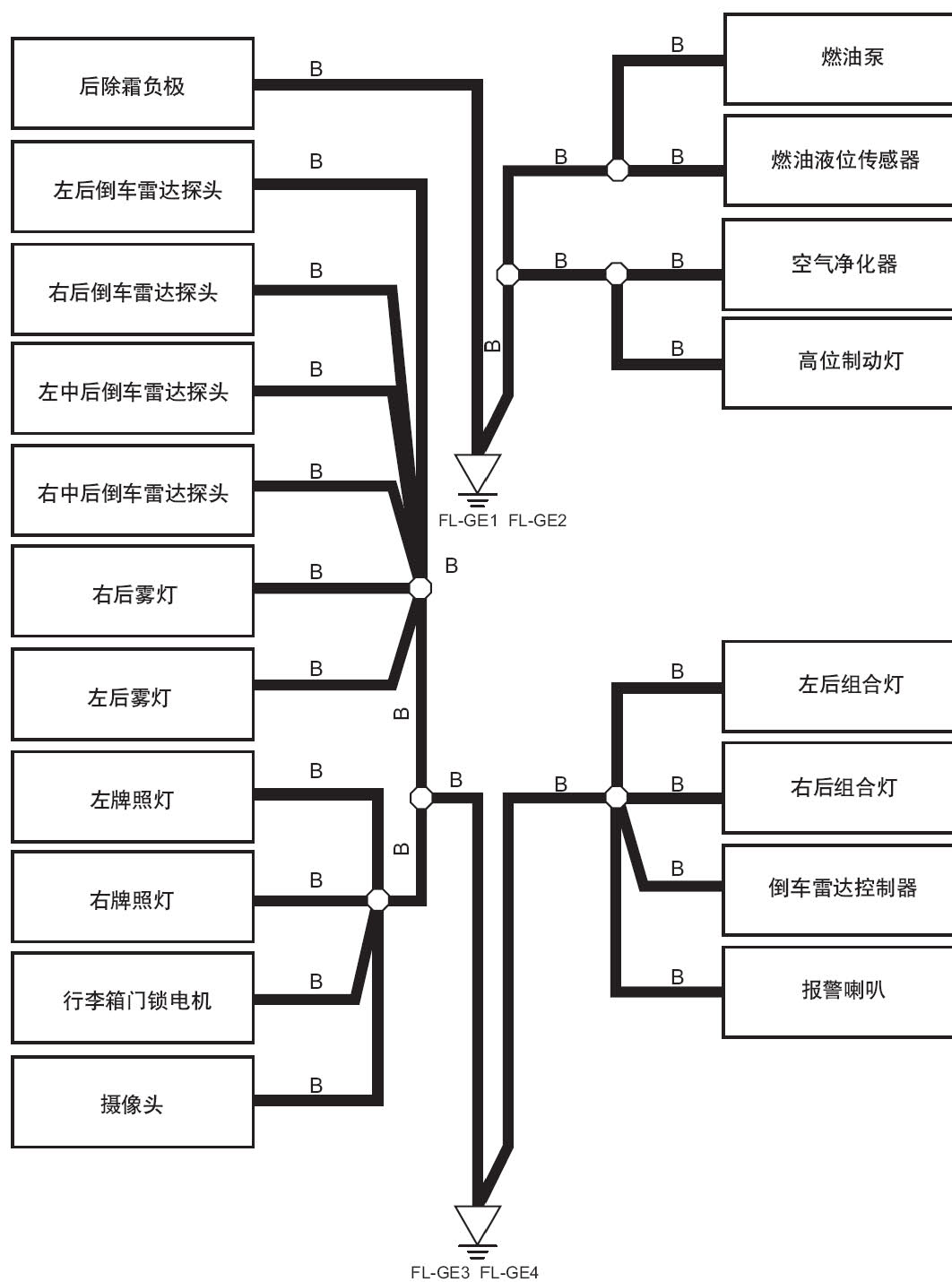
接地线路图7 (FL-GE1, FL-GE2 FL-GE3 FL-GE4)
