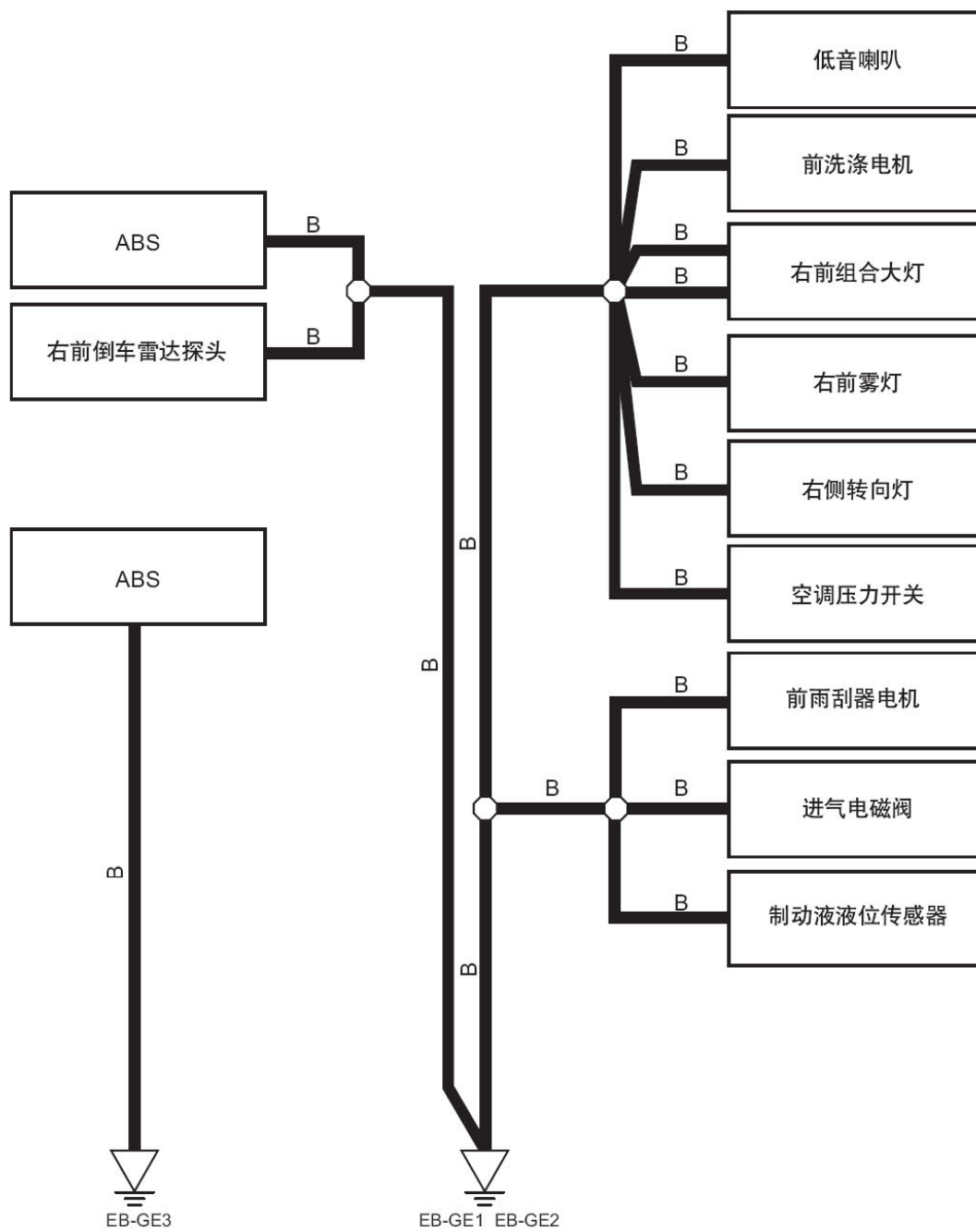
接地线路图2 (EB-GE1, EB-GE2, EB-GE3)
