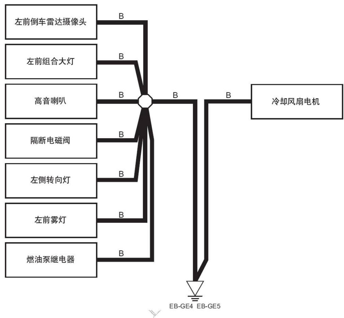
接地线路图3 (EB-GE4, EB-GE5)
