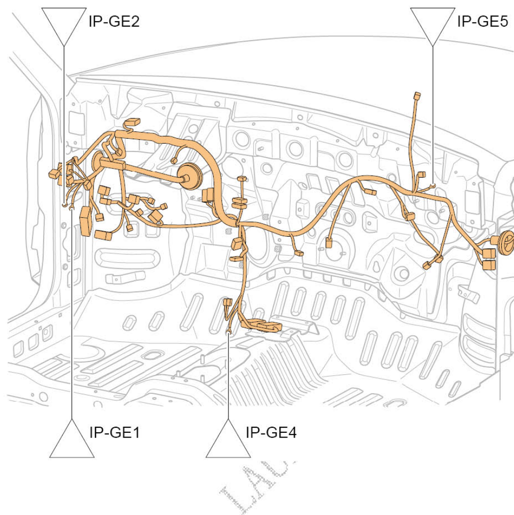
仪表板接地点布置图
