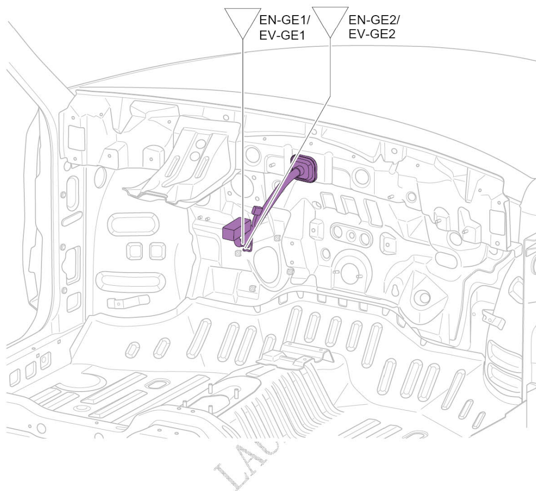
发动机舱接地点布置图（续）
