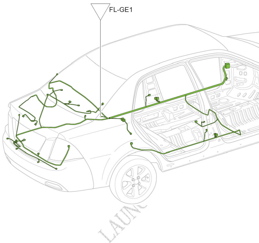
底板接地点布置图
