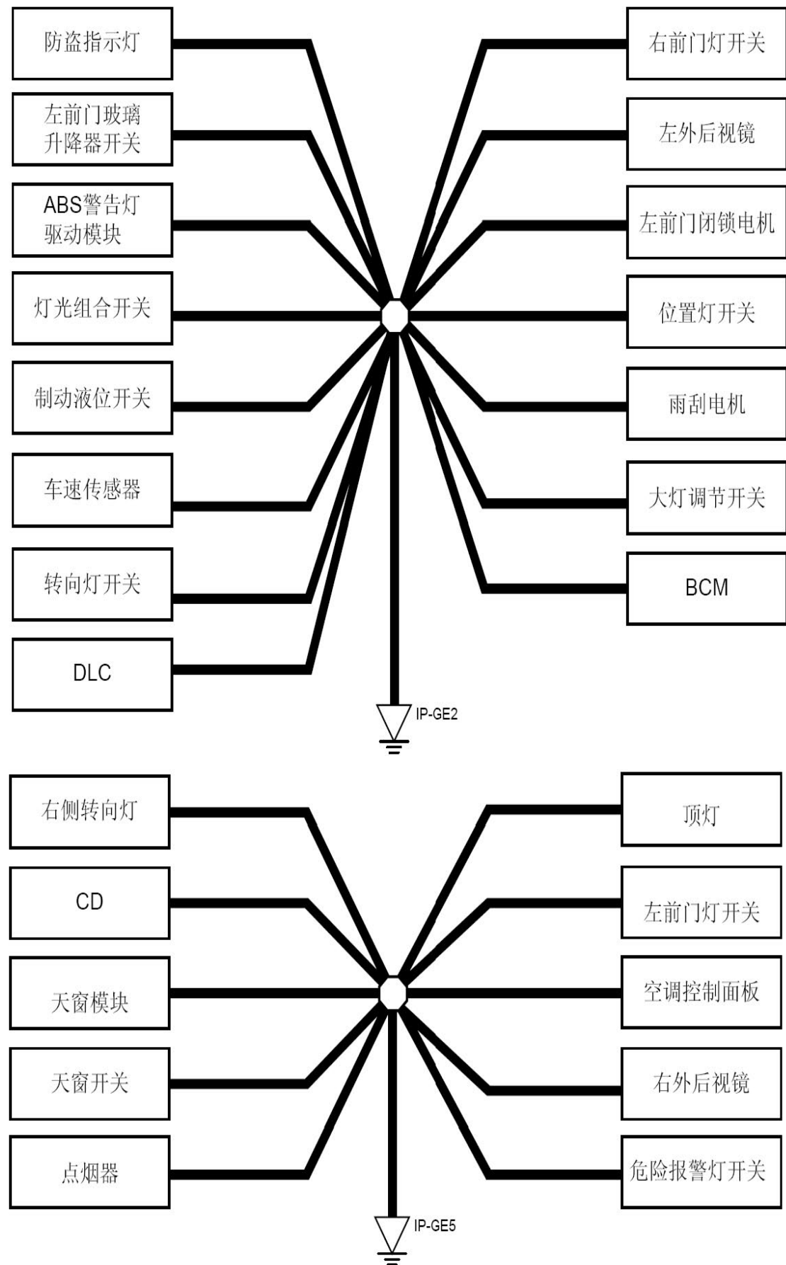
接地线路图4 (IP-GE2、IP-GE5)
