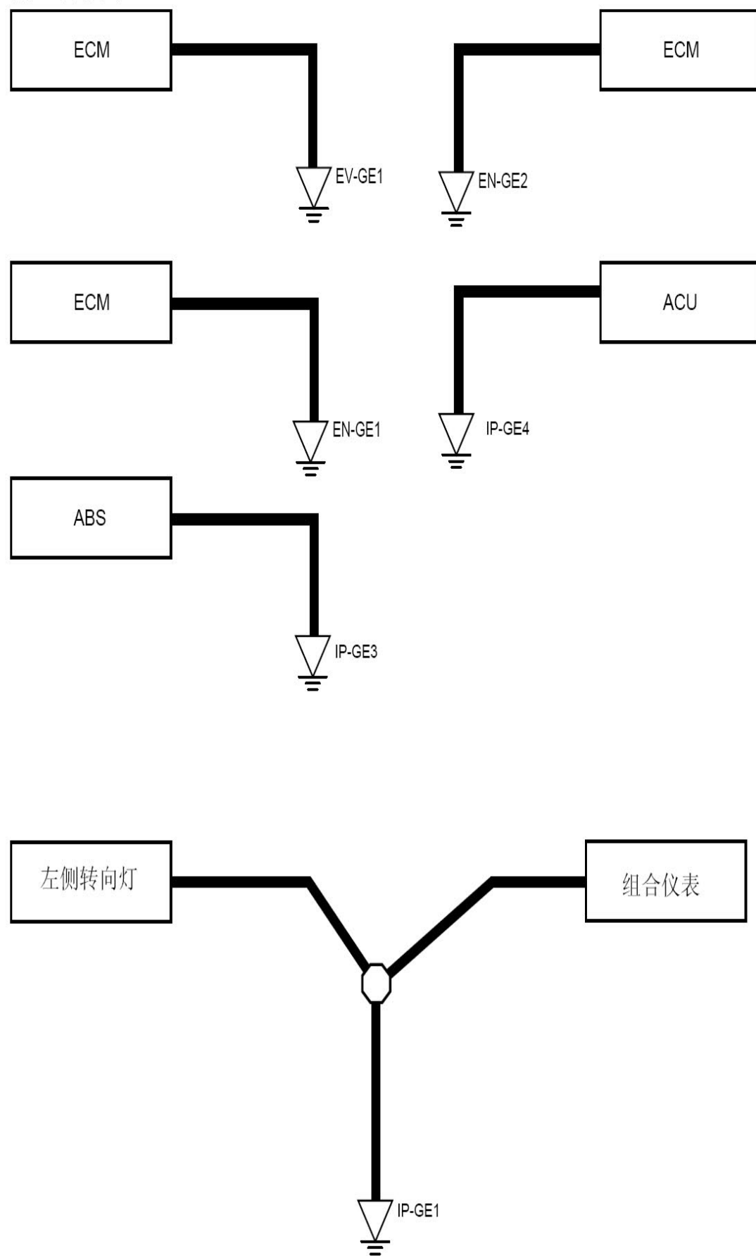
接地线路图3 (EV-GE1、EN-GE1、EN-GE2、IP-GE1、IP-GE3、IP-GE4)
