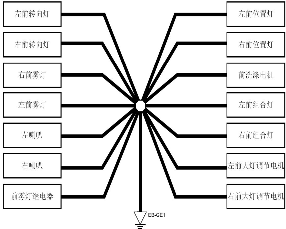
接地线路图1 (EB-GE1、EV-GE2)
