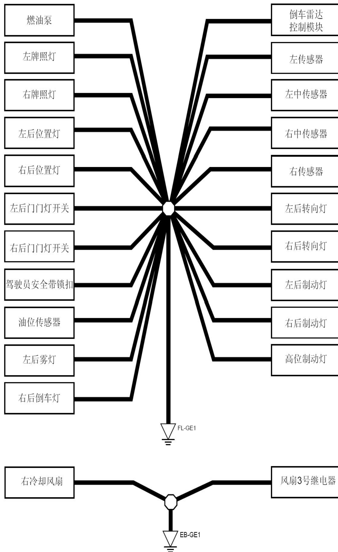
接地线路图2 (FL-GE1、EB-GE1)
