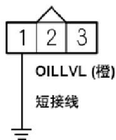
凹头插头导线侧
