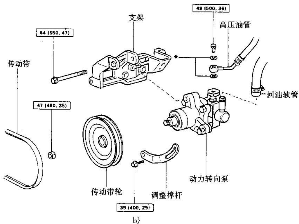
a) 4Y 发动机车型 b) 2L 发动机车型
