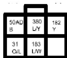
前雨刮器
