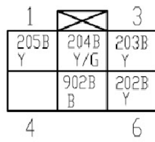
鼓风机开关
