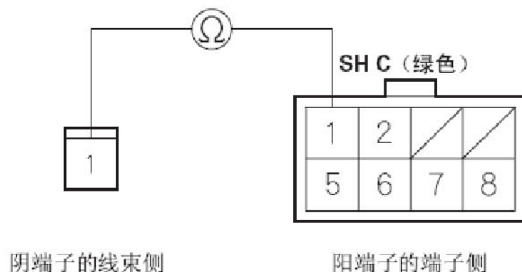
换档电磁阀 C 插接器
