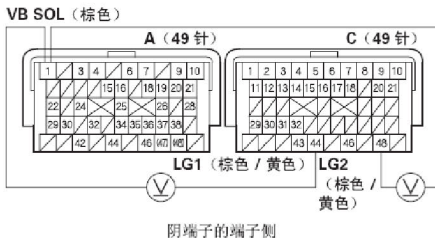
PCM 插接器
