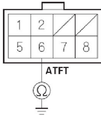
阳端子的端子侧
