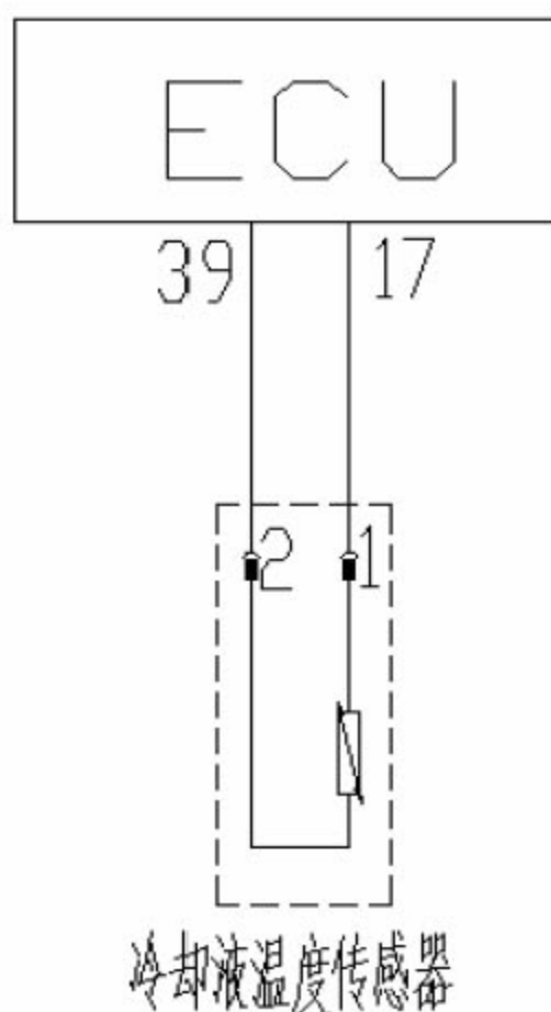
冷却液温度传感器电路图
