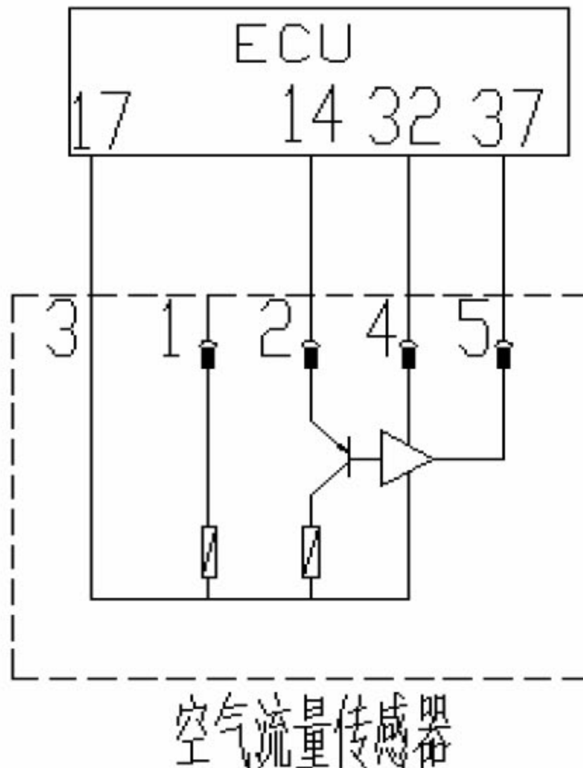
空气流量计电路图
