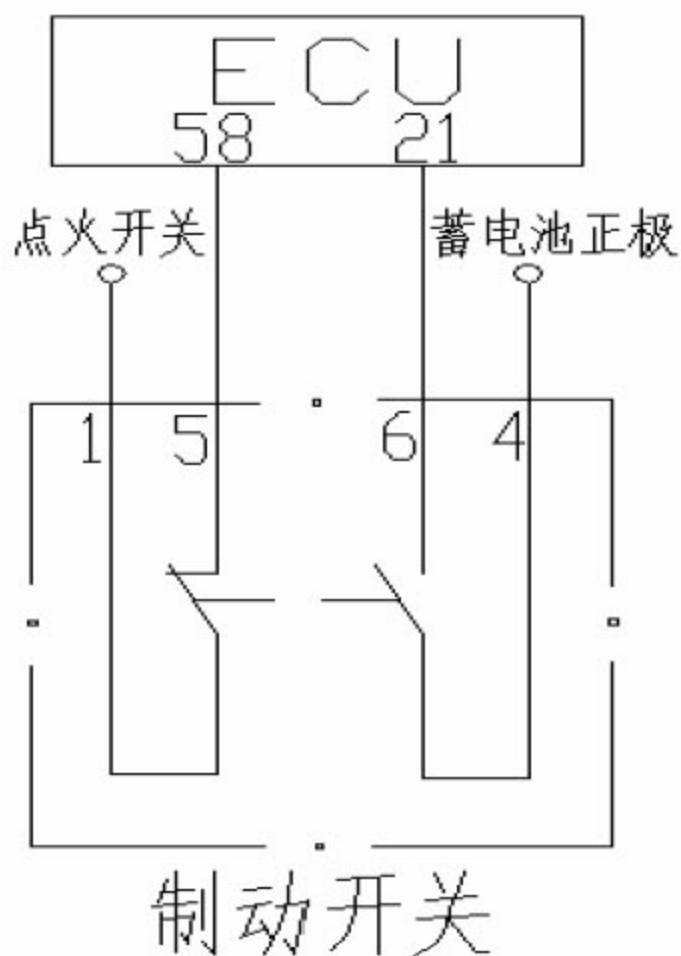
双制动开关电路图
