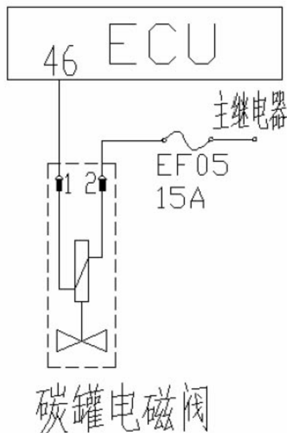
碳罐控制阀电路图
