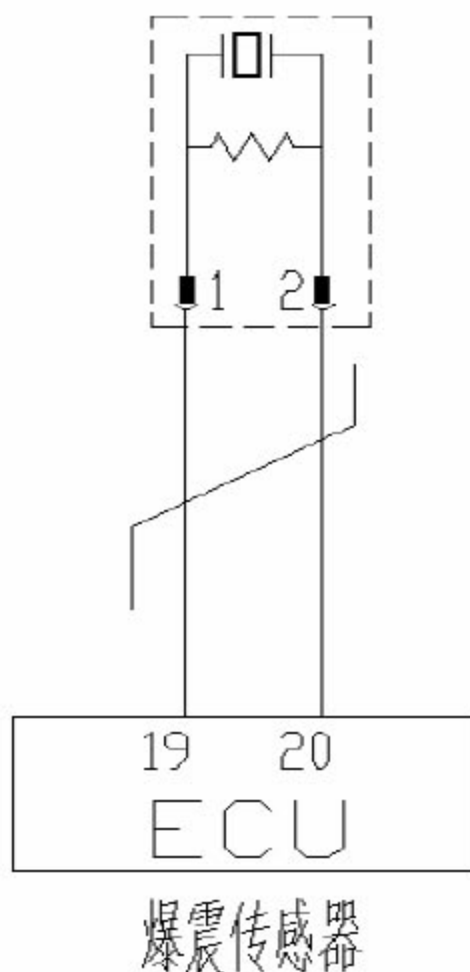
爆震传感器电路图
