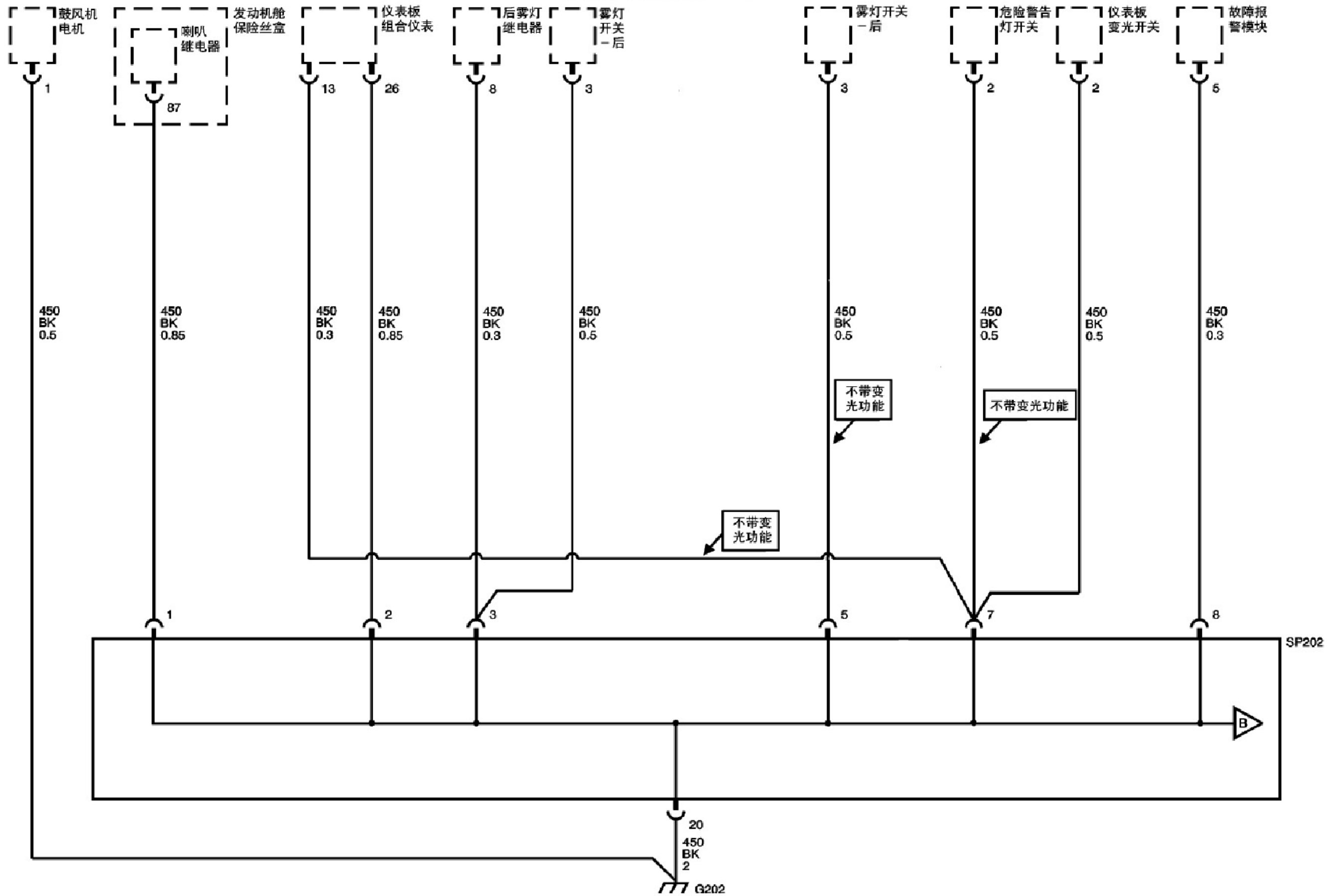
接地分布图(G202 - 1)
