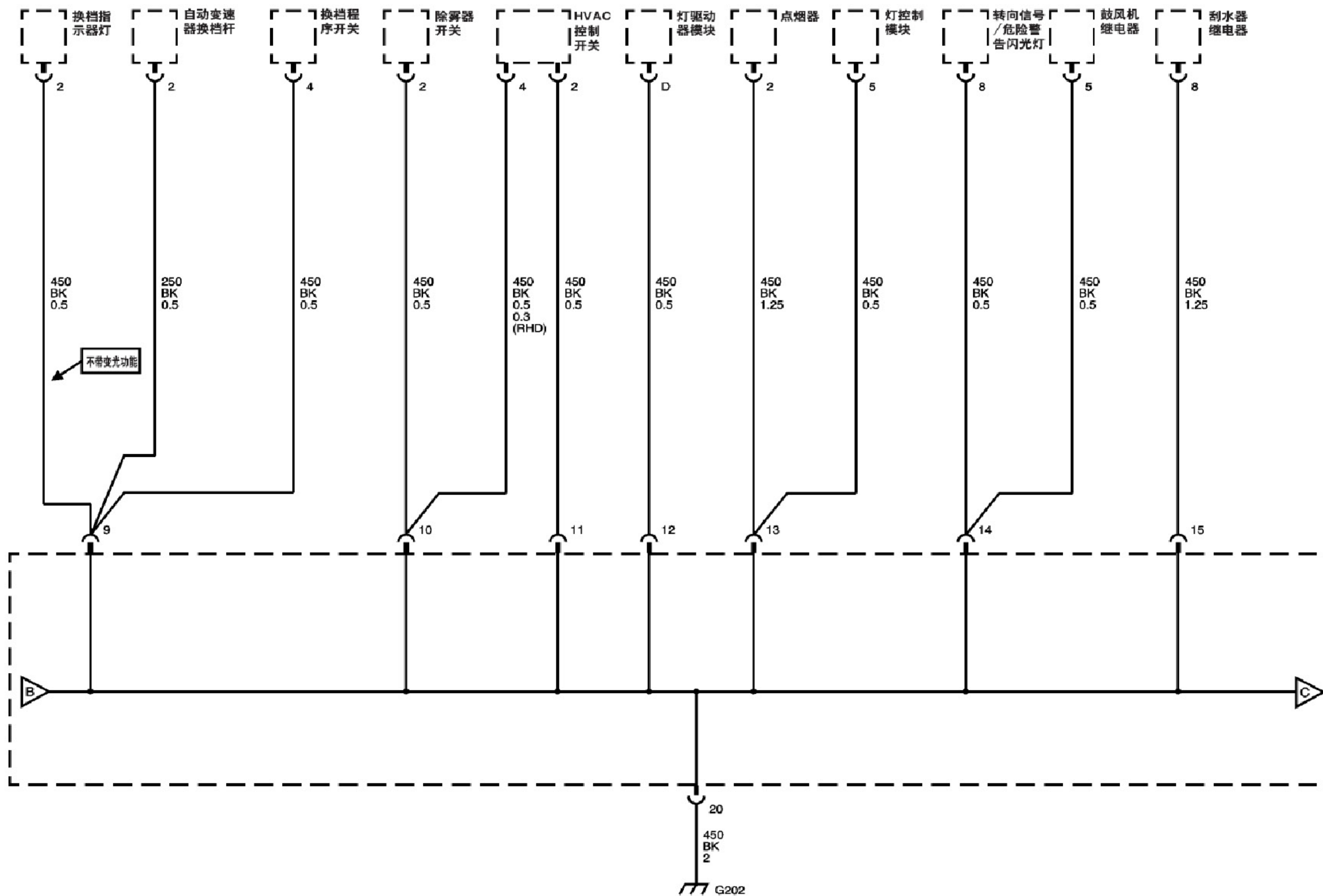
接地分布图(G202 - 2)
