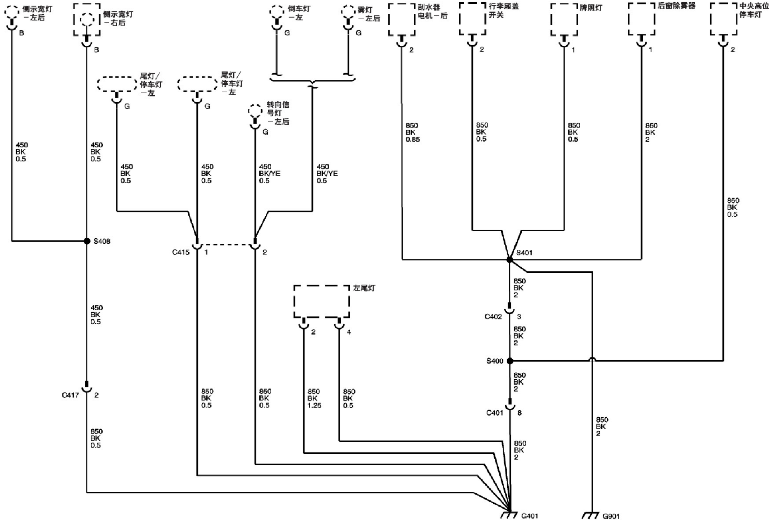
接地分布图 (G402 一两厢车和三厢车)
