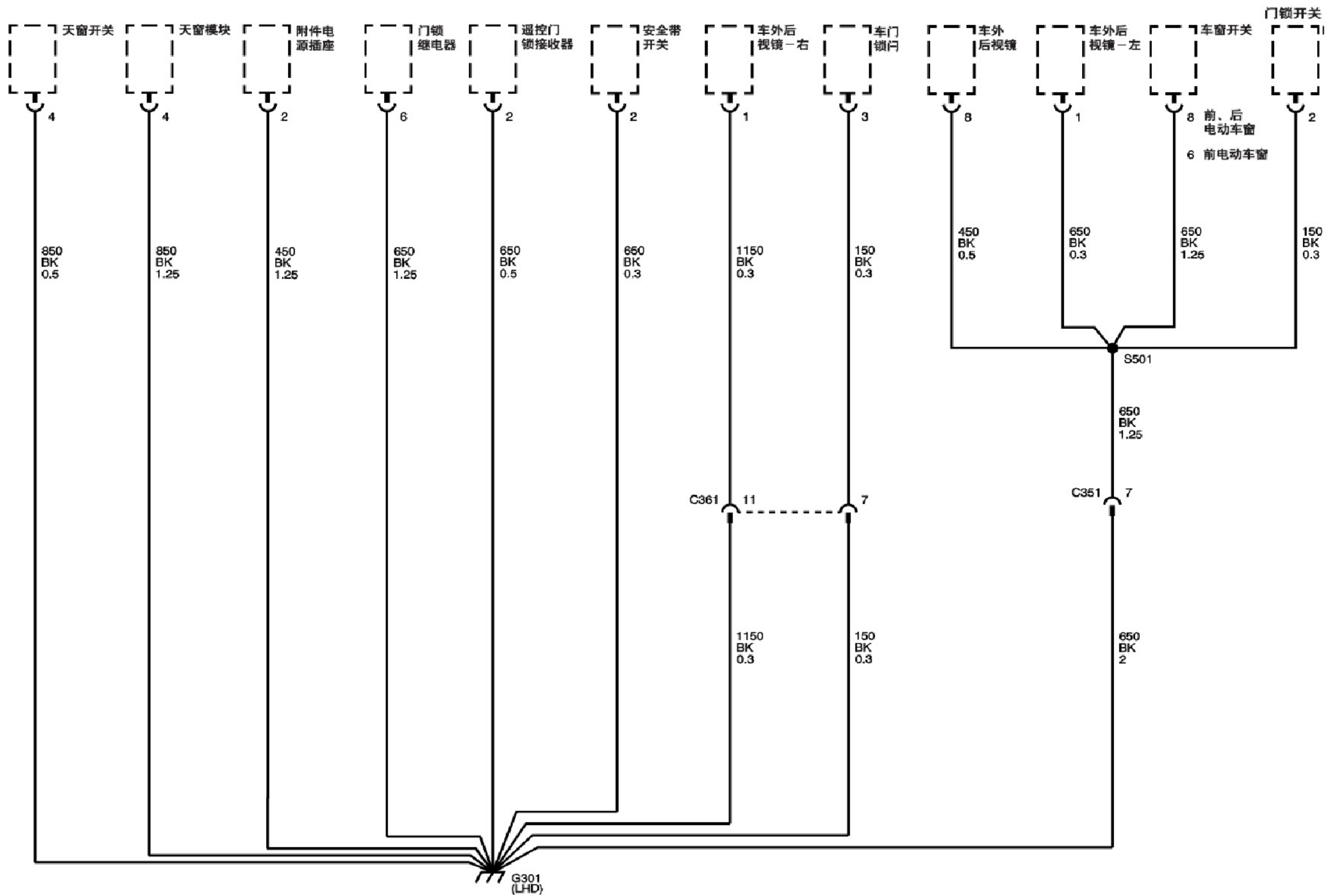
接地分布图 (G301 - 左驾车)
