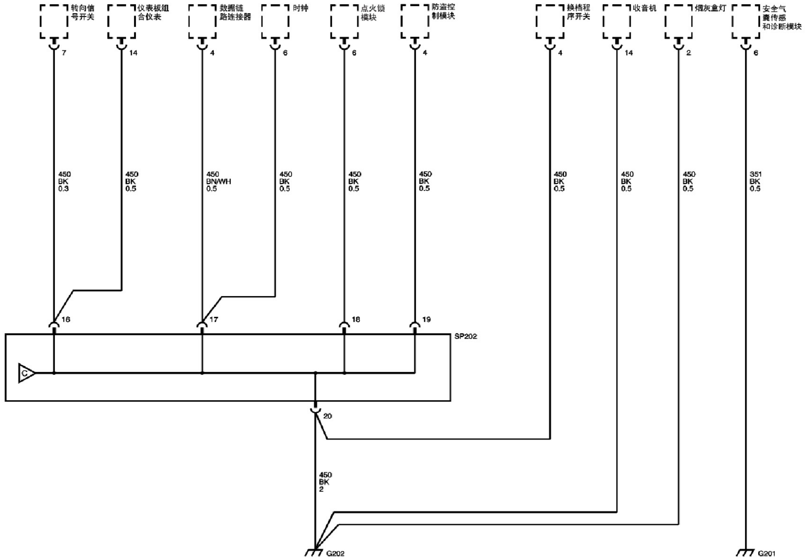
接地分布图 (G201 和 G202 - 3)
