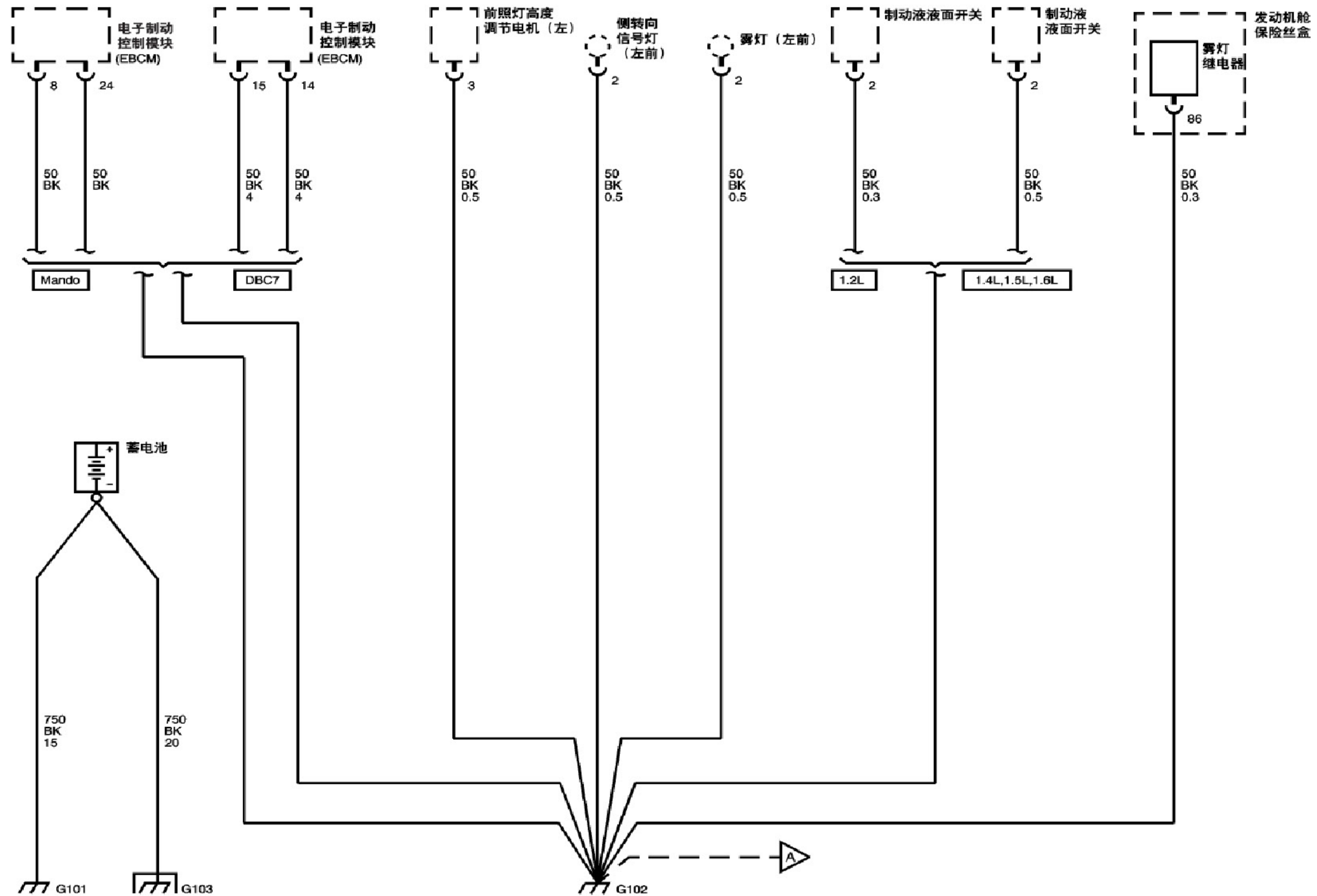
接地分布图 (G101、G102 和 G103)
