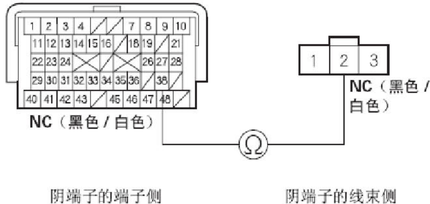
输出轴（副轴） 转速传感器插接器
