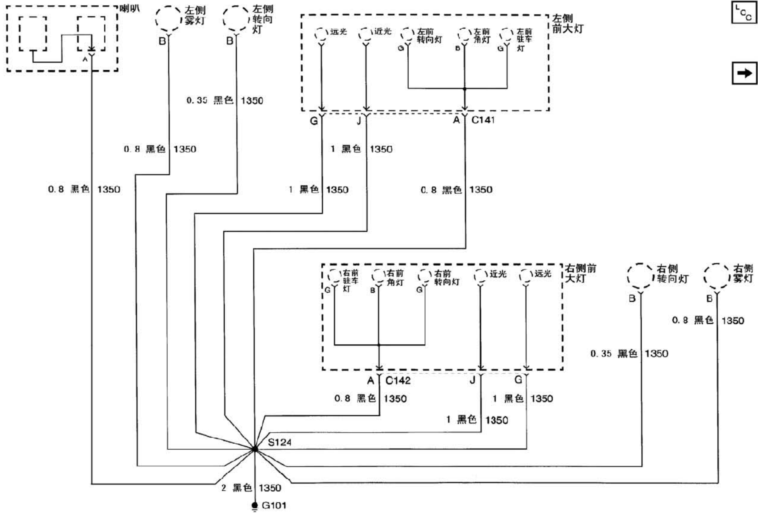
接地分配图 (G101)
