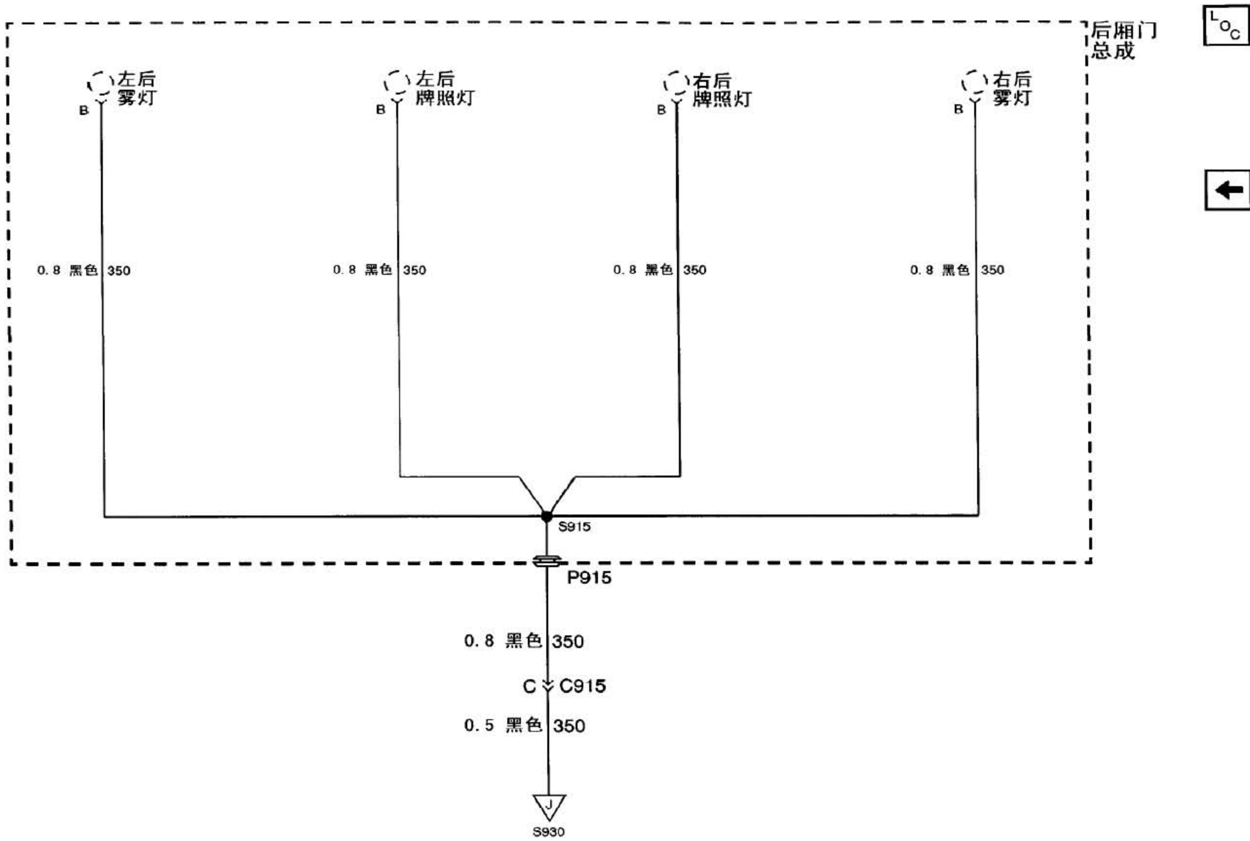
接地分配图 (G402)
