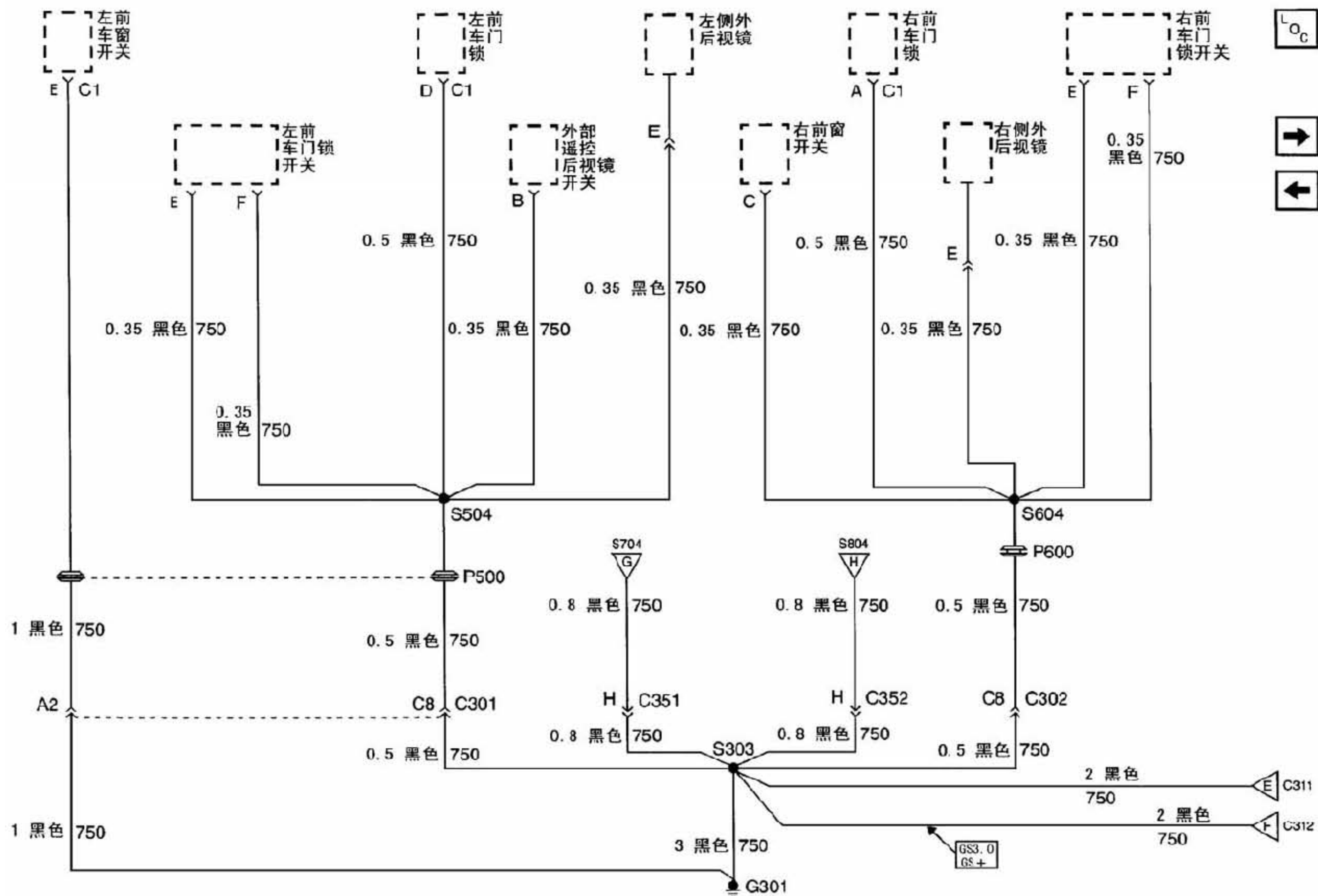
接地分配图 (G301, 3之1)
