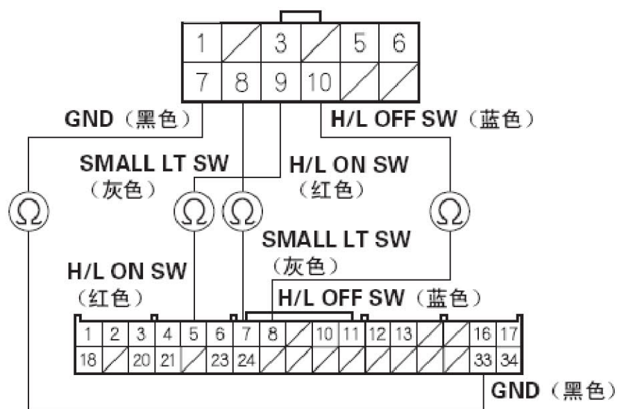
仪表板下保险丝 / 继电器盒插接器 M (34 针) 阴端子的线束侧
