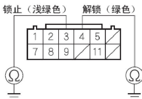
阴端子的线束侧
