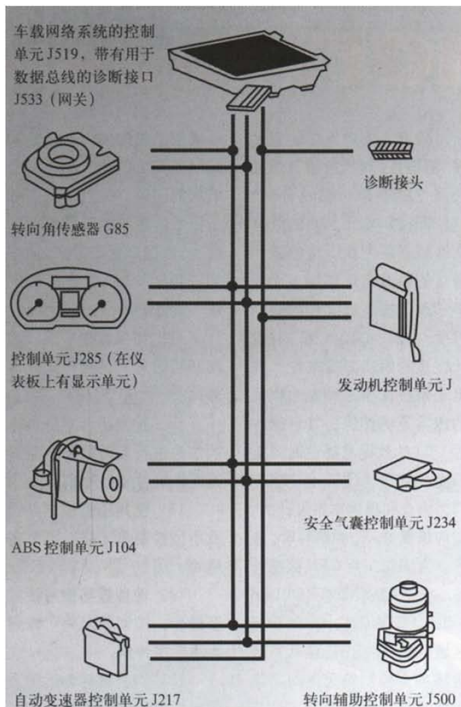
图 5 汽车 CAN 驱动装置数据总线系统的组成
