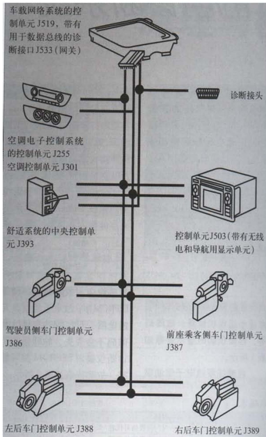
图 6 CAN 舒适模式数据总线系统的组成
