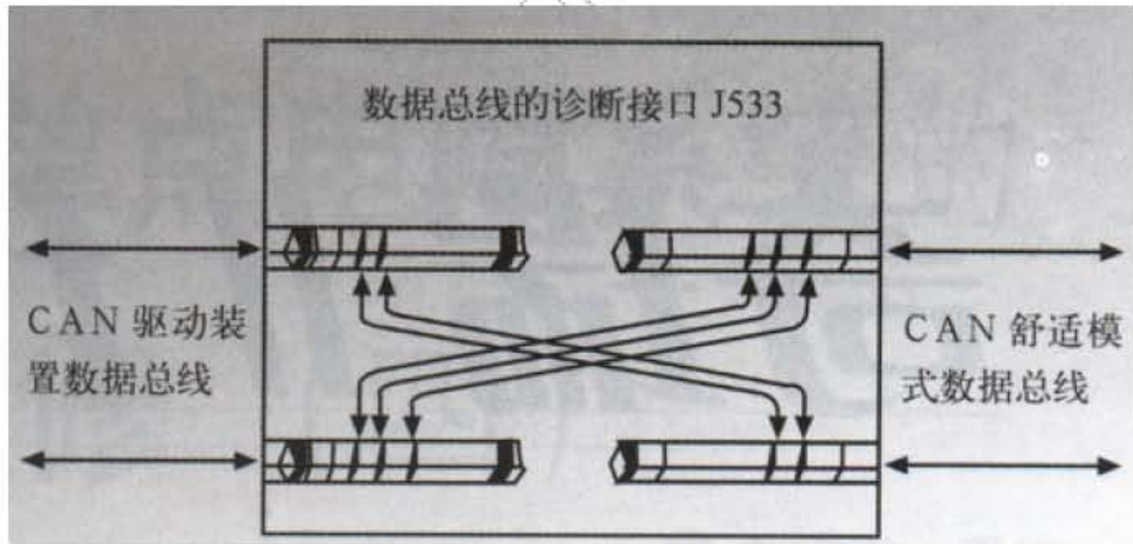
图 8 CAN 驱动装置数据总线和 CAN 舒适模式数据总线间进行数据交换
