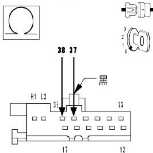
变速器控制 模块 C2 (NAG1)
