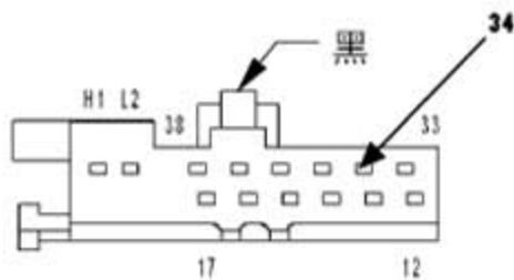
变速器控制 模块 C2 (NAG1)
