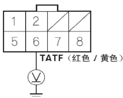
阴端子的线束侧
