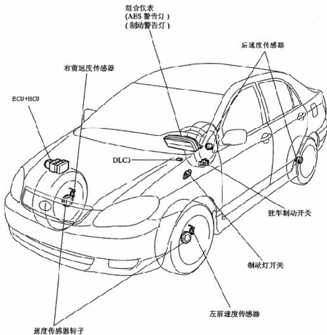
防抱死制动系统位置布置图 (2)
