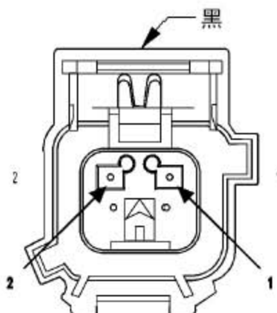
发动机冷却液 温度传感器
