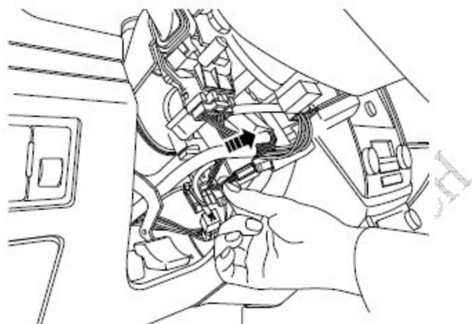
B). 连接发动机电子防盗线圈线束连接器。
