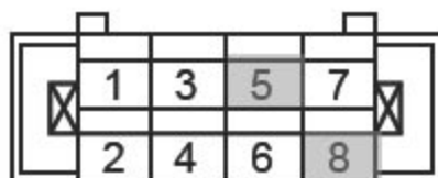
发动机防盗单元1线束连接器 IP25
