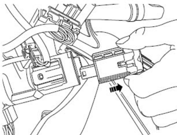
H). 拆卸发动机电子防盗线圈。
