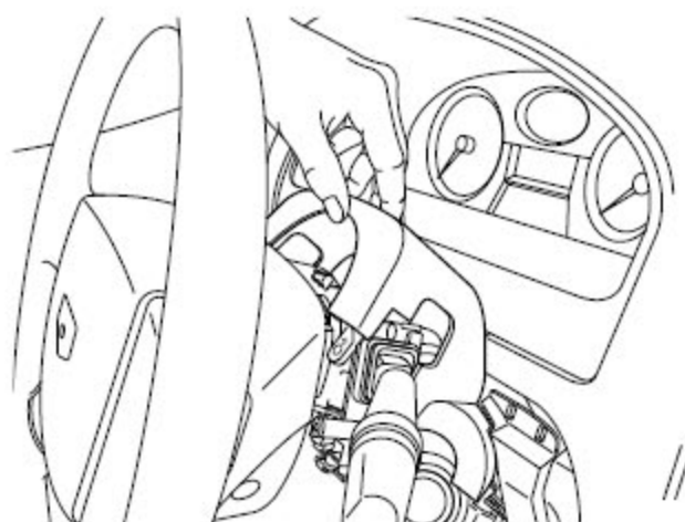
C). 安装转向柱上护板。
