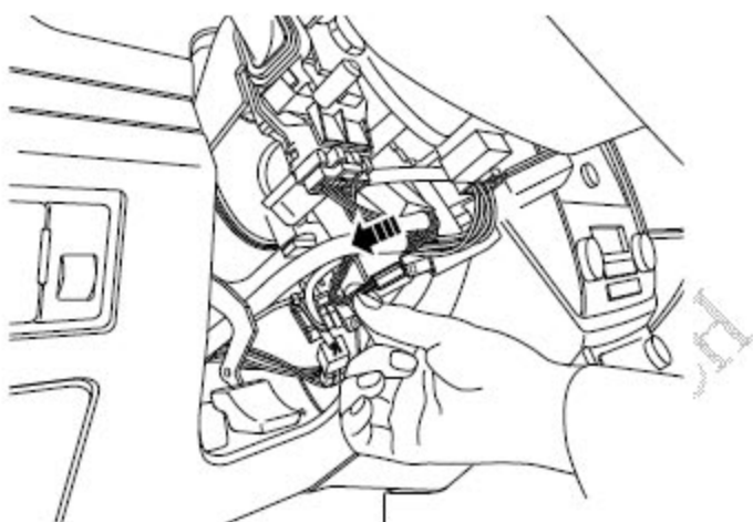
G). 断开发动机电子防盗线圈线束连接器。
