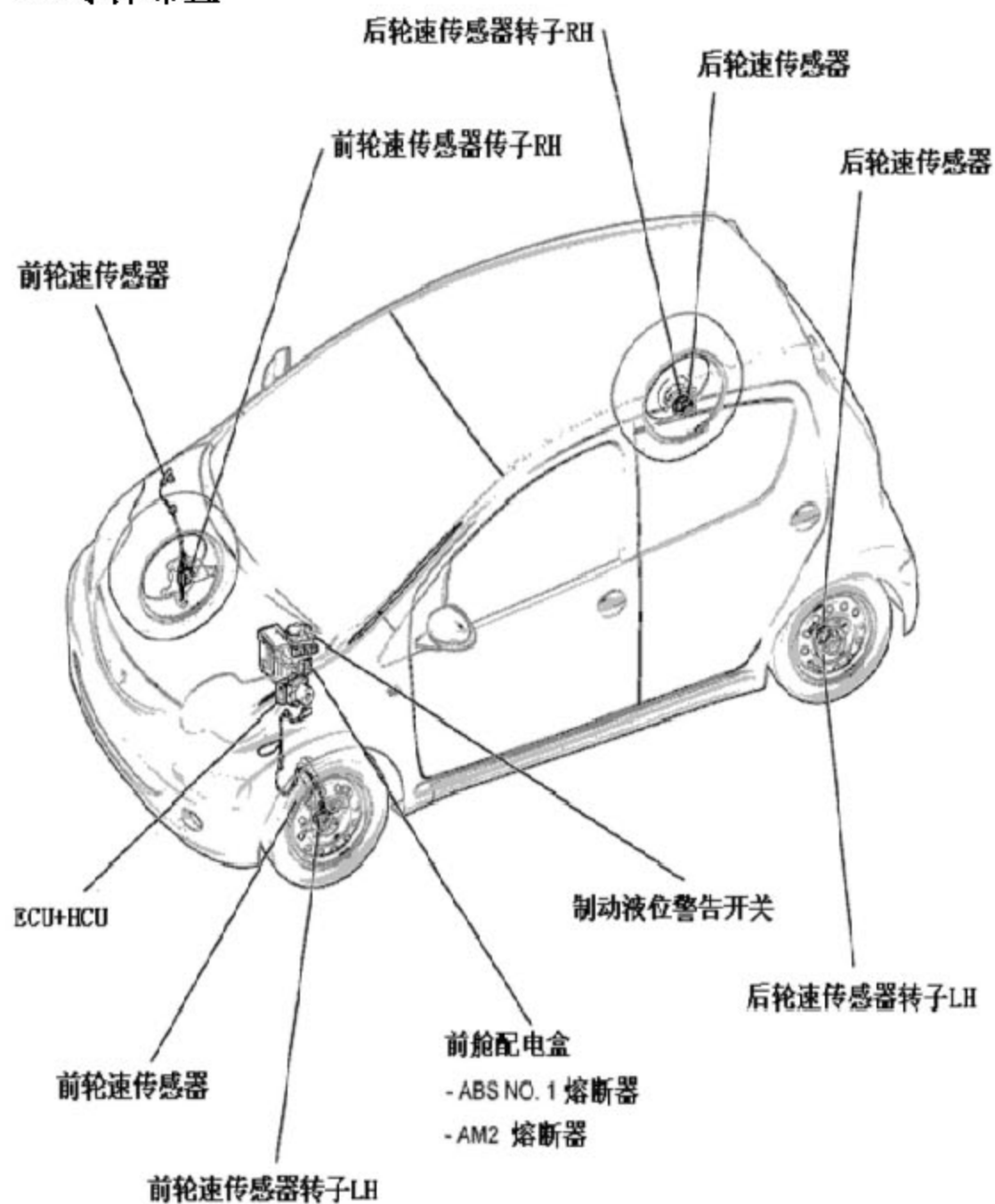
防抱死制动系统布置图 1
