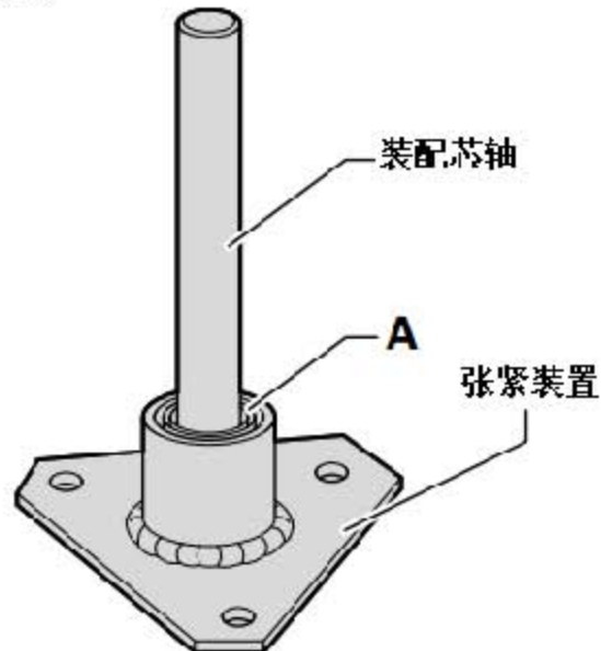
图 2 将径向止推球轴承的内圈(下图 A 所示)压入外圈, 内圈(下图 A 所示)必须用外圈卡紧
