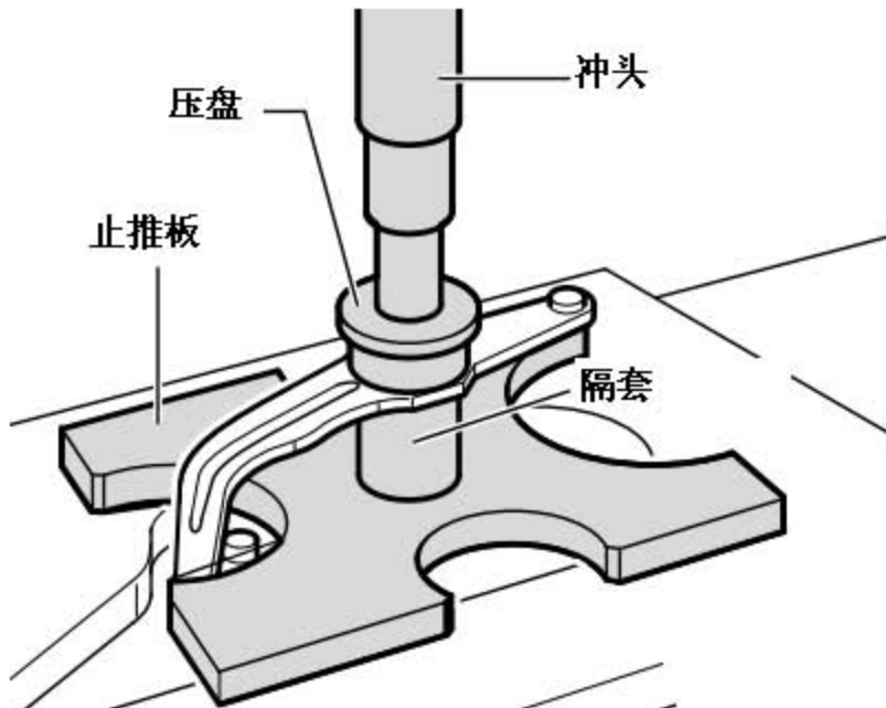
图 4 拆卸弹簧垫圈
