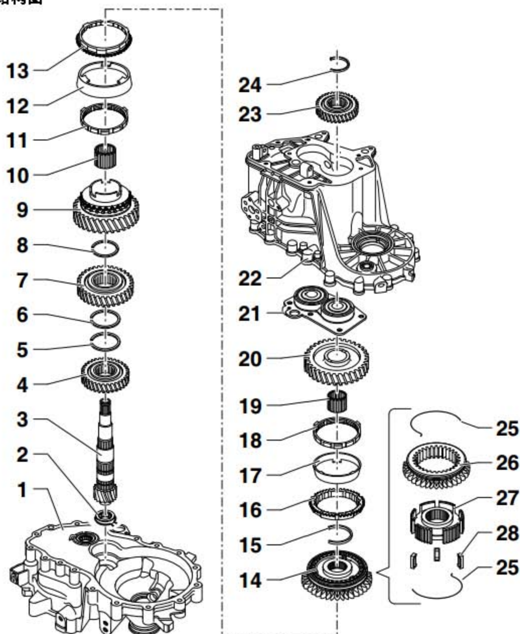
结构图
