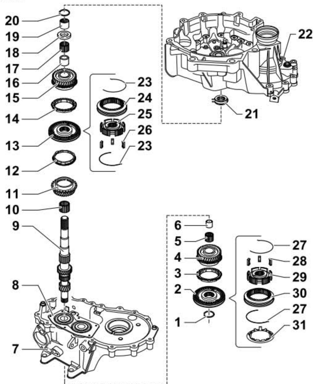
结构图
