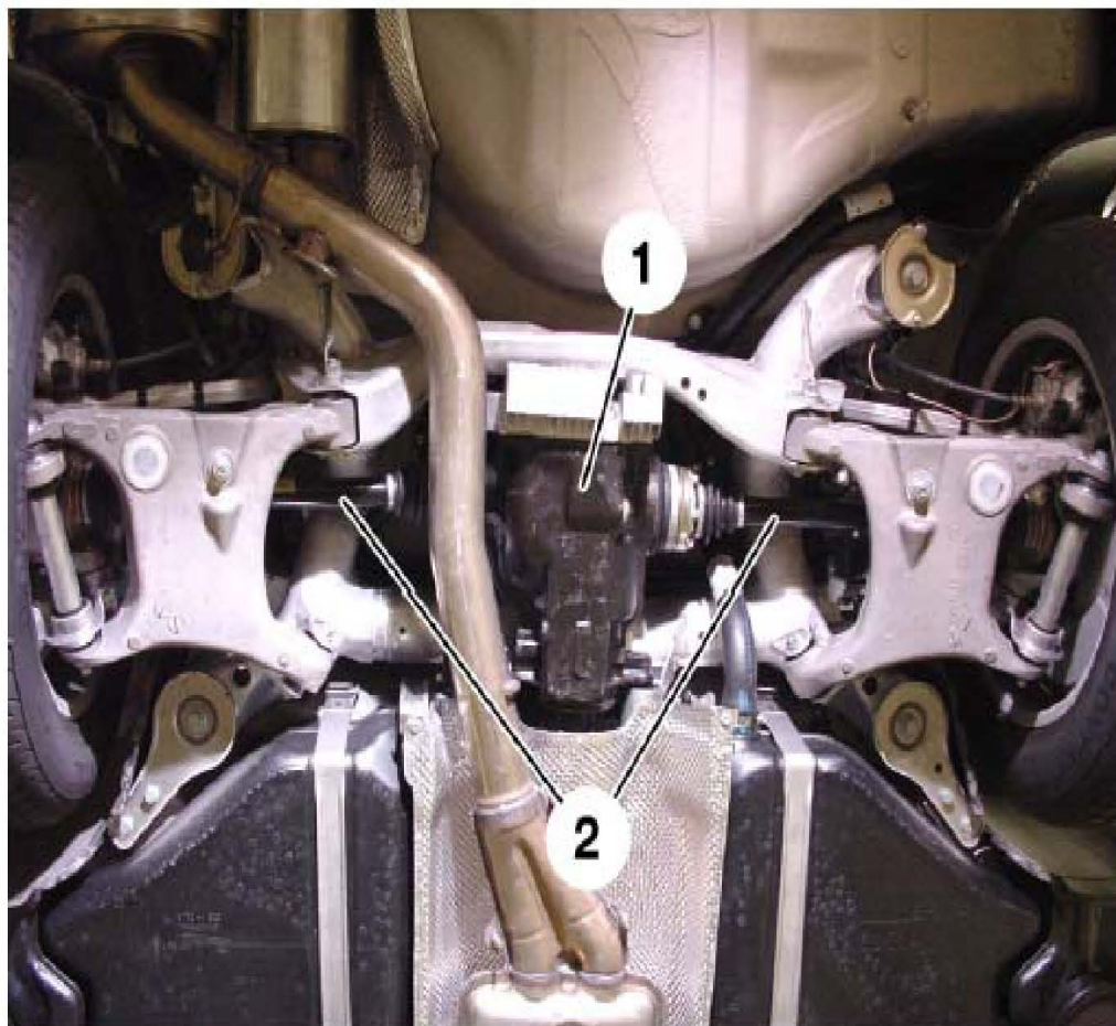
主减速器
