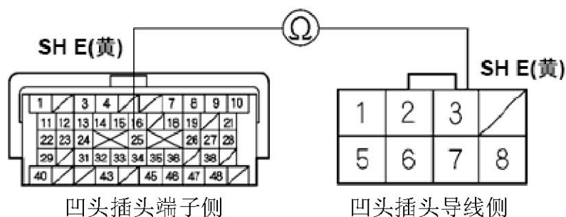
PCM插头B(49芯)
